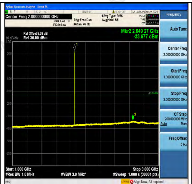
GPRS1900-512-0-1000~3000MHz-PASS
