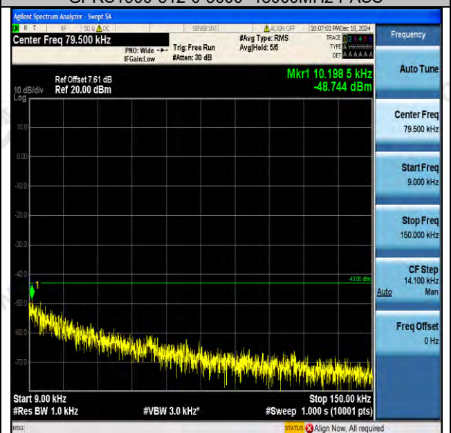
GPRS1900-661-0-0.009~0.15MHz-PASS
