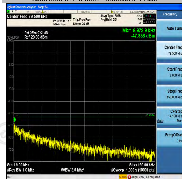
GSM1900-661-0-0.009~0.15MHz-PASS
