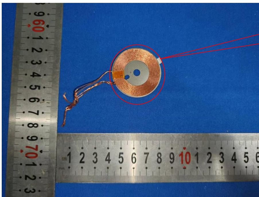
Phone ANT1
