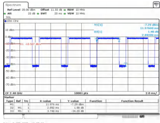
\pi/4 DQPSK(2-DH5)_Channel 78
