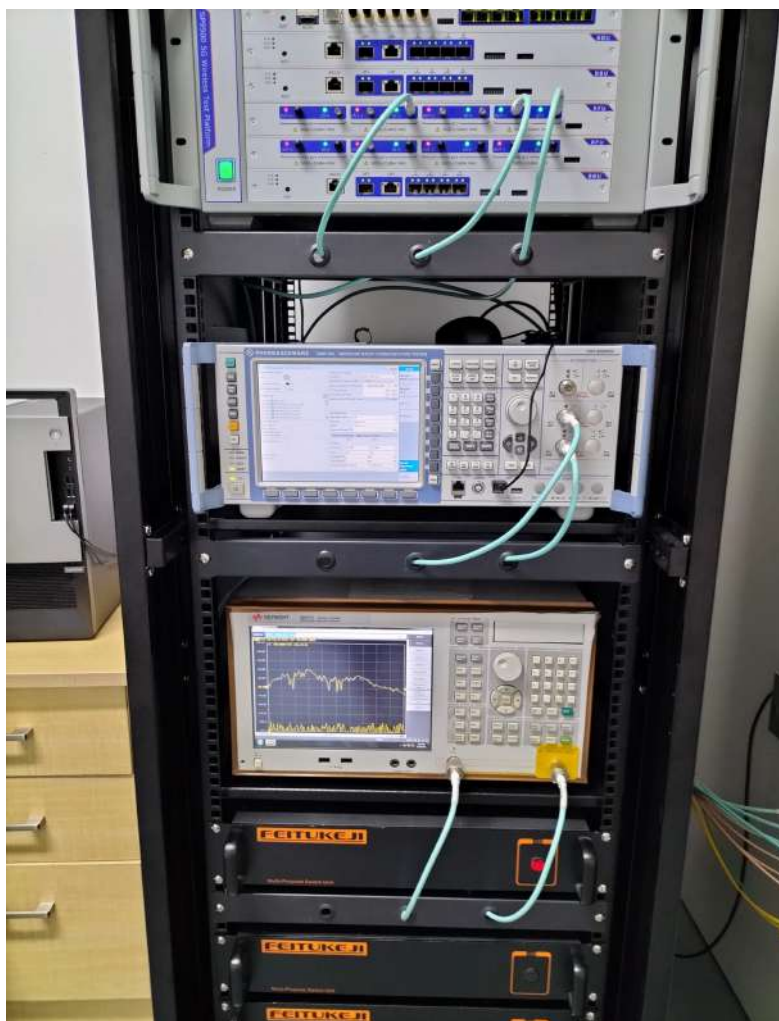
测试设备
