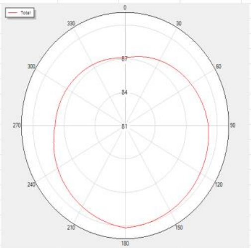
BLUETOOTH_Tis_Rssi_H39 Total
