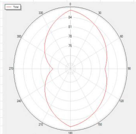
BLUETOOTH_Tis_Rssi_V78 Total
