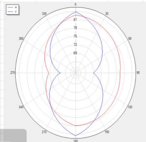
BLUETOOTH_Tis_Rssi_V78 Polar
