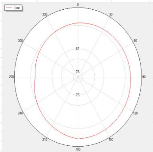
BLUETOOTH_Tis_Rssi_V0 Total
