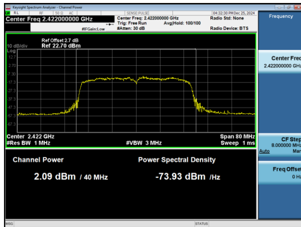
802.11n(HT40) ANT 1
