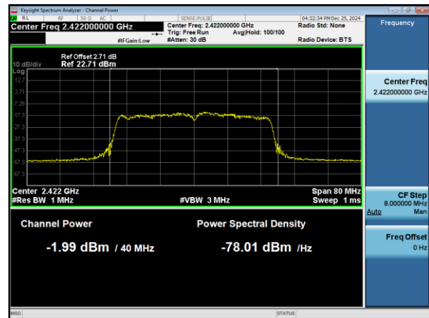
802.11n(HT40) ANT 2
