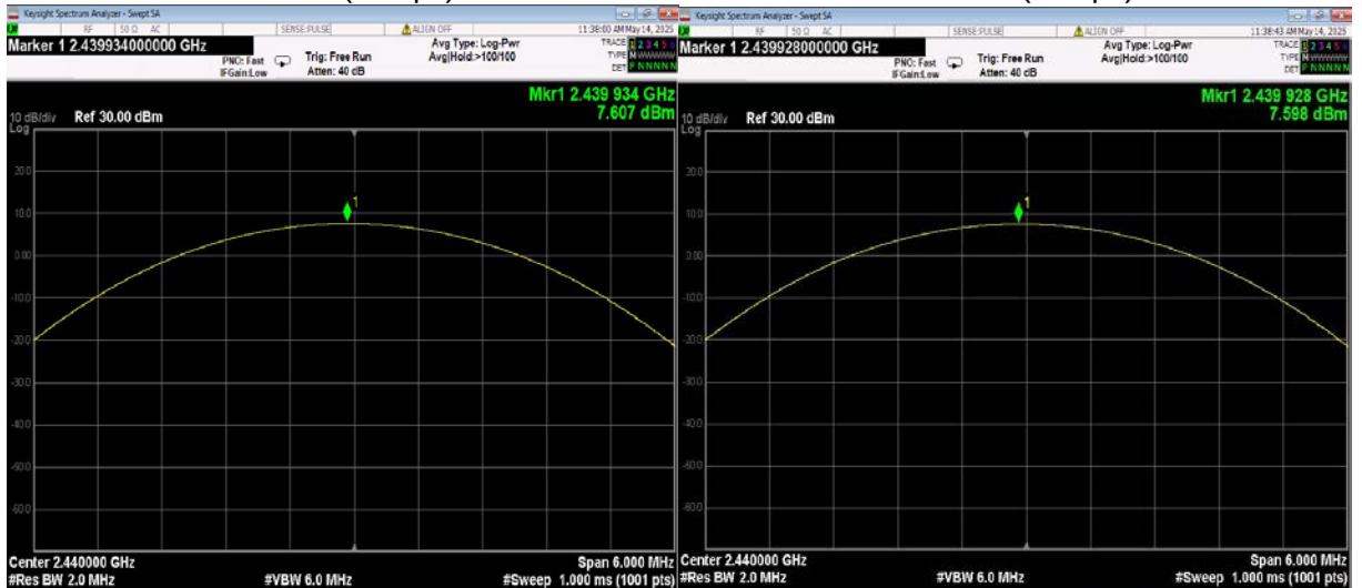
2440MHz(1Mbps)
