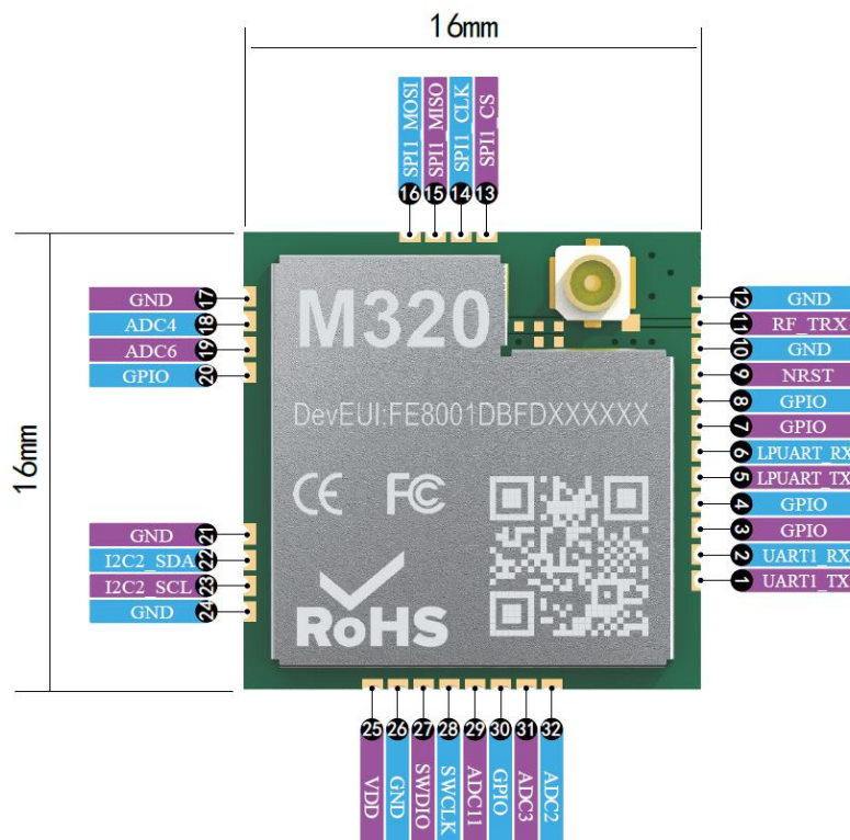
图 2-1 引脚分布图
