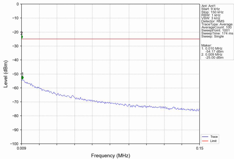
Band41_15MHz_QPSK_MCH_2593MHz_RB_1_0 NTN
