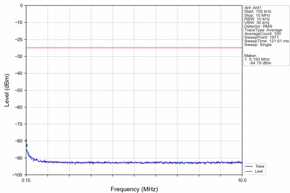
Band41_15MHz_QPSK_MCH_2593MHz_RB_1_0 NTN
