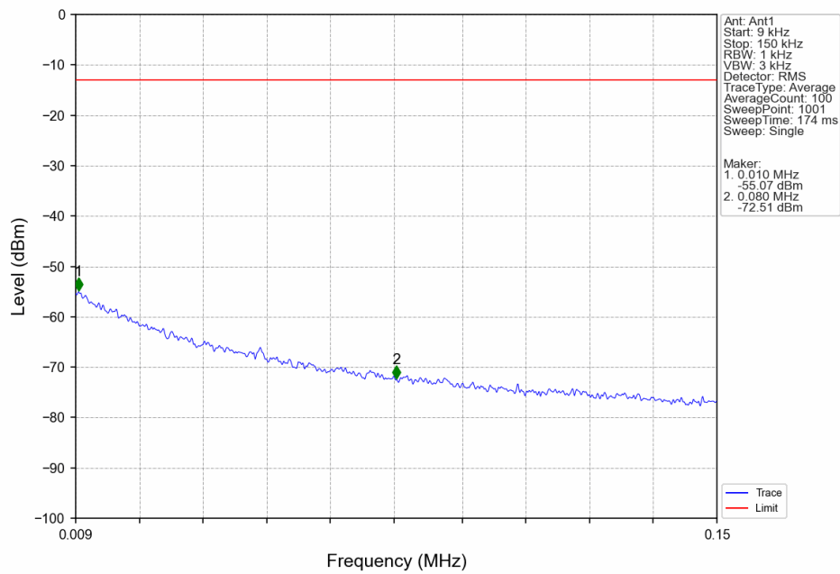
Band26b 5MHz QPSK LCH 826.5MHz RB 1 0 NTN
