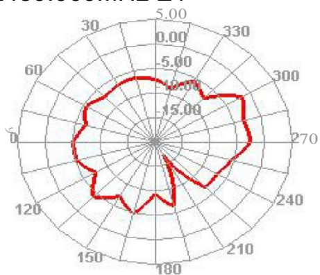
2450.000MHz E1
