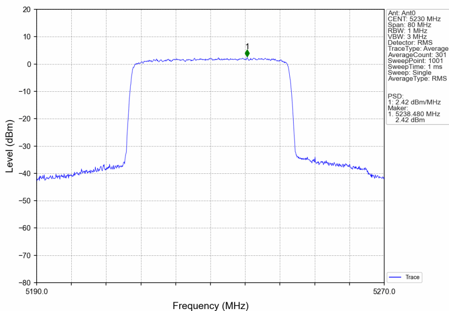
40M_HCH_5230MHz_Ant0_NTNV
