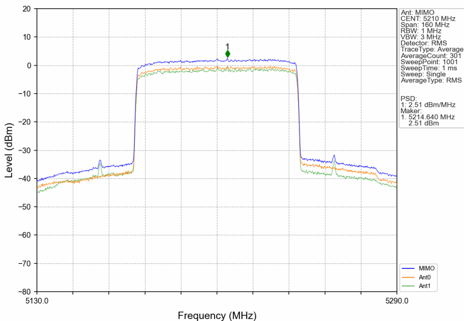
80M_HCH_5210MHz_MIMO_NTNV
