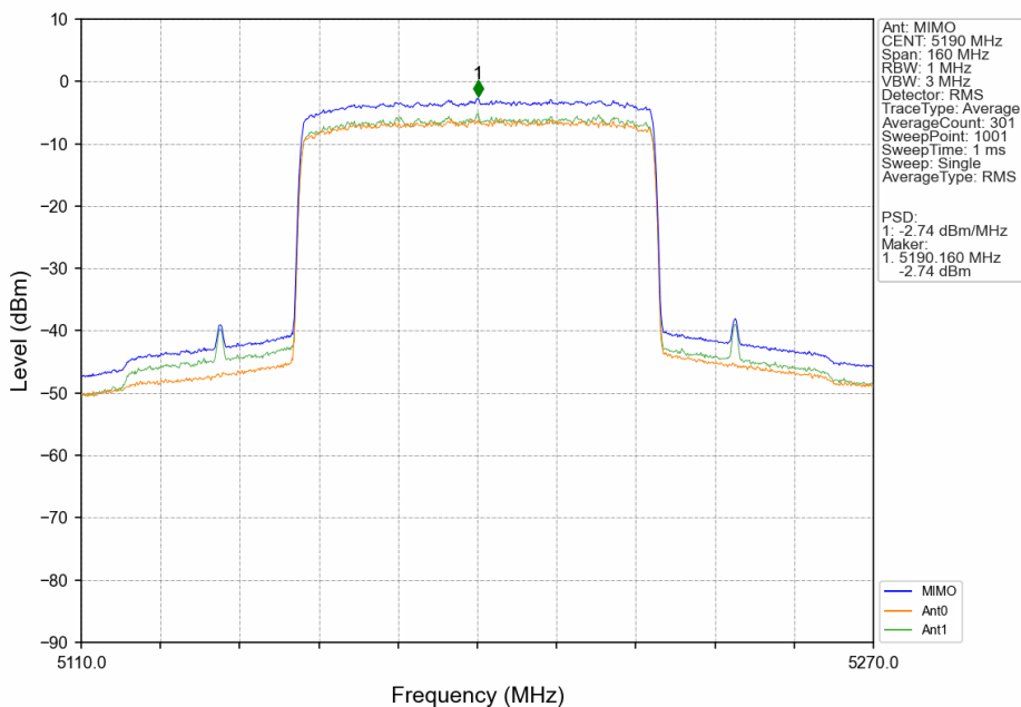
80M_LCH_5190MHz_MIMO_NTNV
