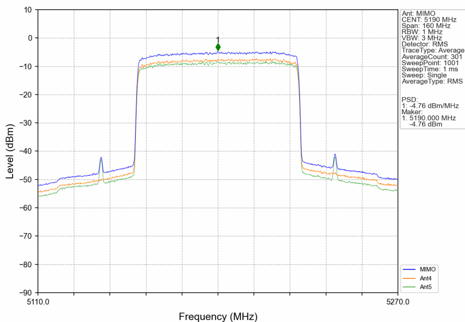
80M_LCH_5190MHz_MIMO_NTNV
