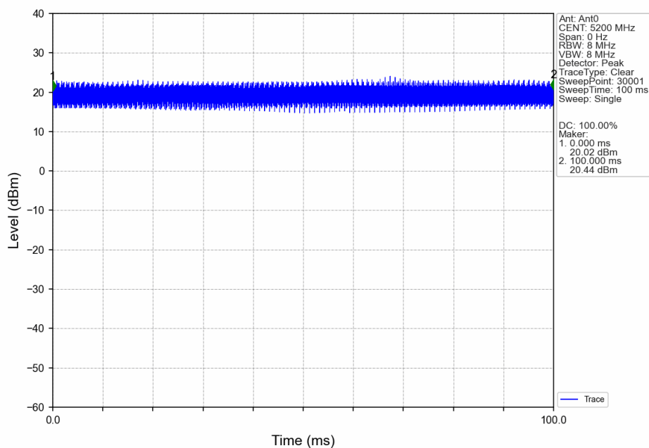
20M_MCH_5200MHz_Ant0_NTNV
