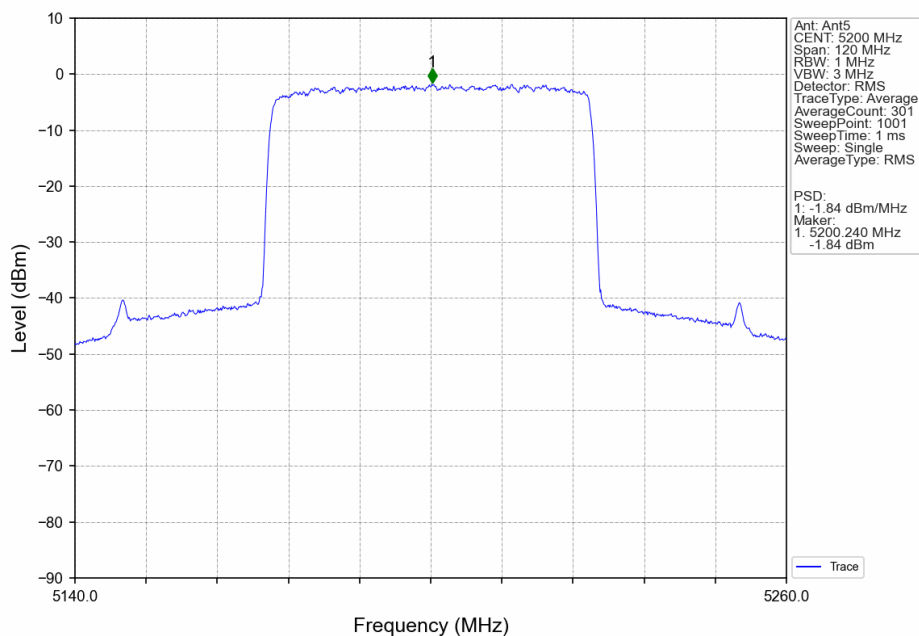
60M_MCH_5200MHz_MIMO_NTNV
