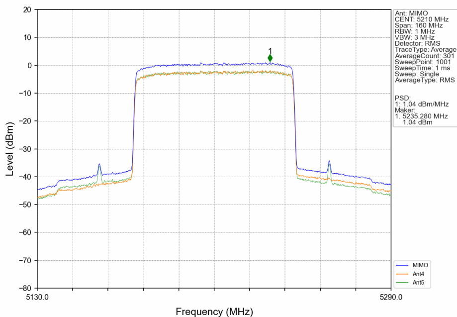
80M_HCH_5210MHz_MIMO_NTNV
