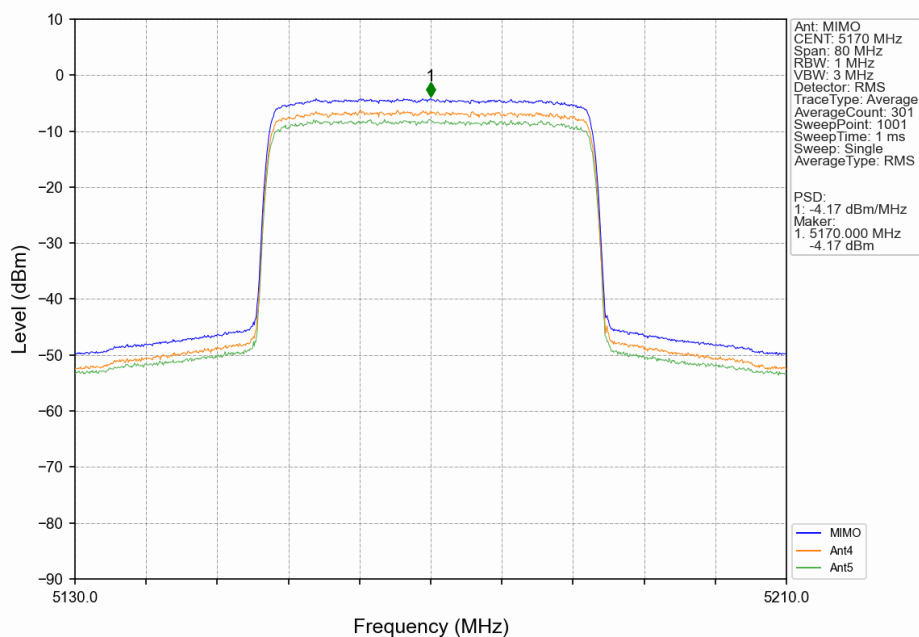
40M_LCH_5170MHz_MIMO_NTNV
