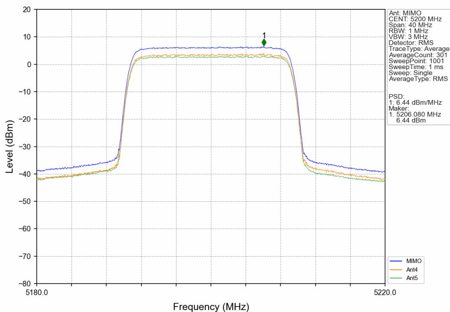
20M_MCH_5200MHz_MIMO_NTNV
