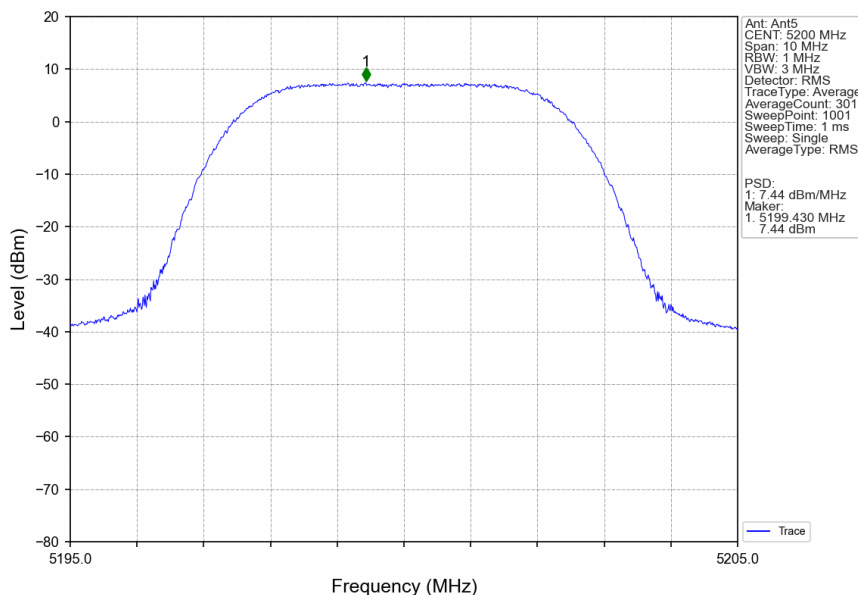
5M_MCH_5200MHz_MIMO_NTNV
