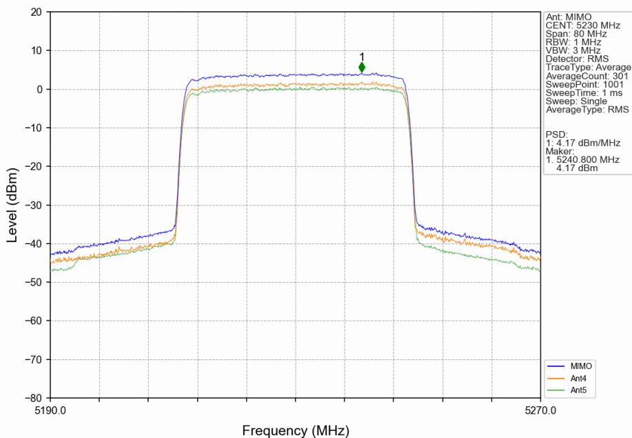
40M_HCH_5230MHz_MIMO_NTNV
