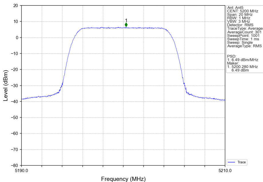
10M_MCH_5200MHz_Ant5_NTNV
