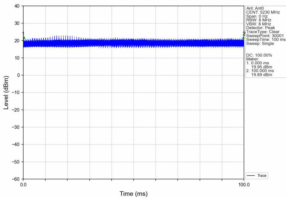
40M_HCH_5230MHz_Ant0_NTNV
