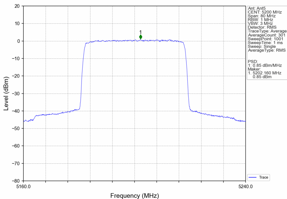
40M_MCH_5200MHz_Ant5_NTNV
