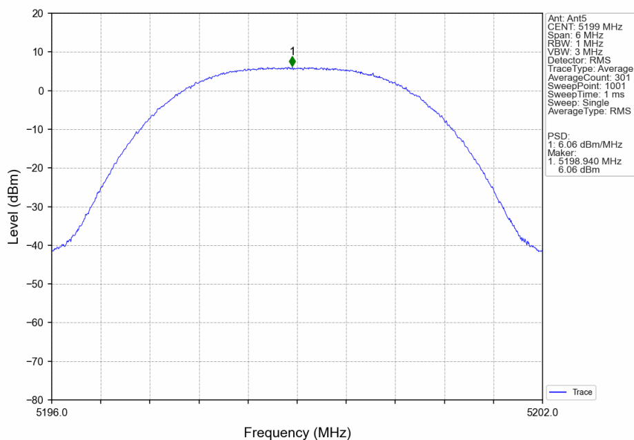
3M_MCH_5199MHz_Ant5_NTNV
