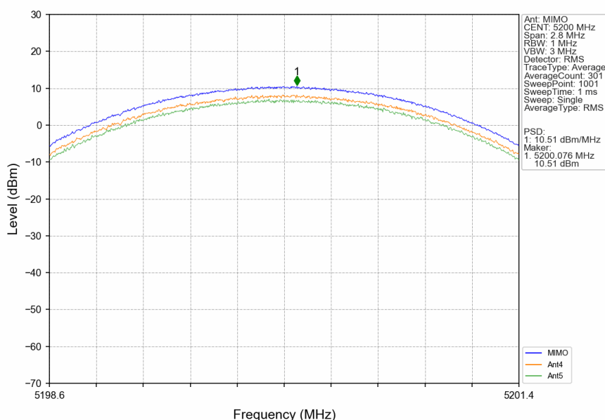
1.4M_MCH_5200MHz_MIMO_NTNV
