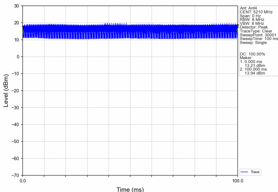
80M_HCH_5210MHz_Ant4_NTNV
