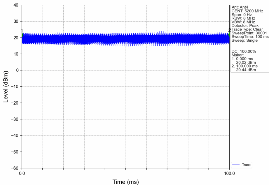
20M_MCH_5200MHz_Ant4_NTNV
