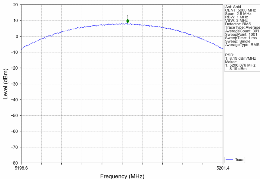
1.4M_MCH_5200MHz_Ant4_NTNV
