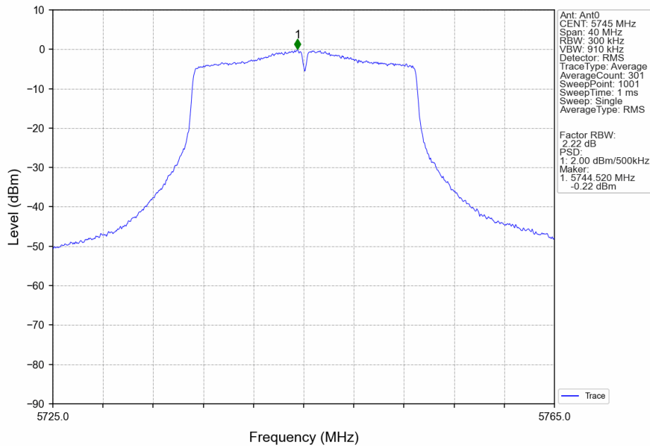
802.11ac(VHT20)_LCH_5745MHz_Ant0_NTNV
