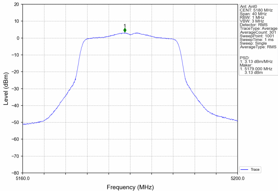
802.11ac(VHT20)_LCH_5180MHz_Ant0_NTNV
