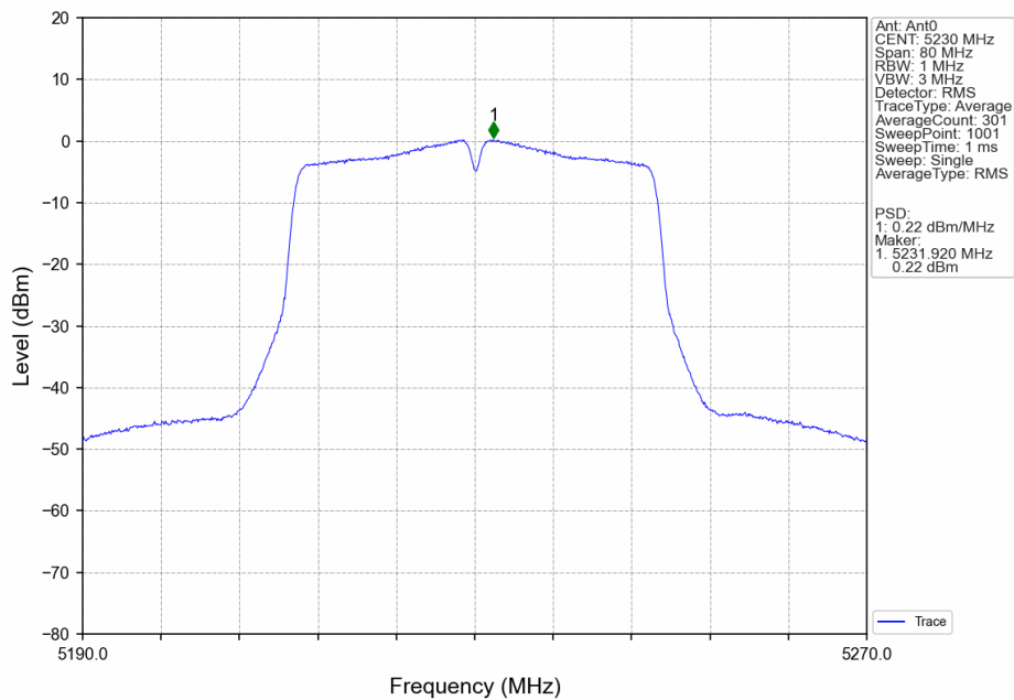
802.11ac(VHT40)_HCH_5230MHz_Ant0_NTNV
