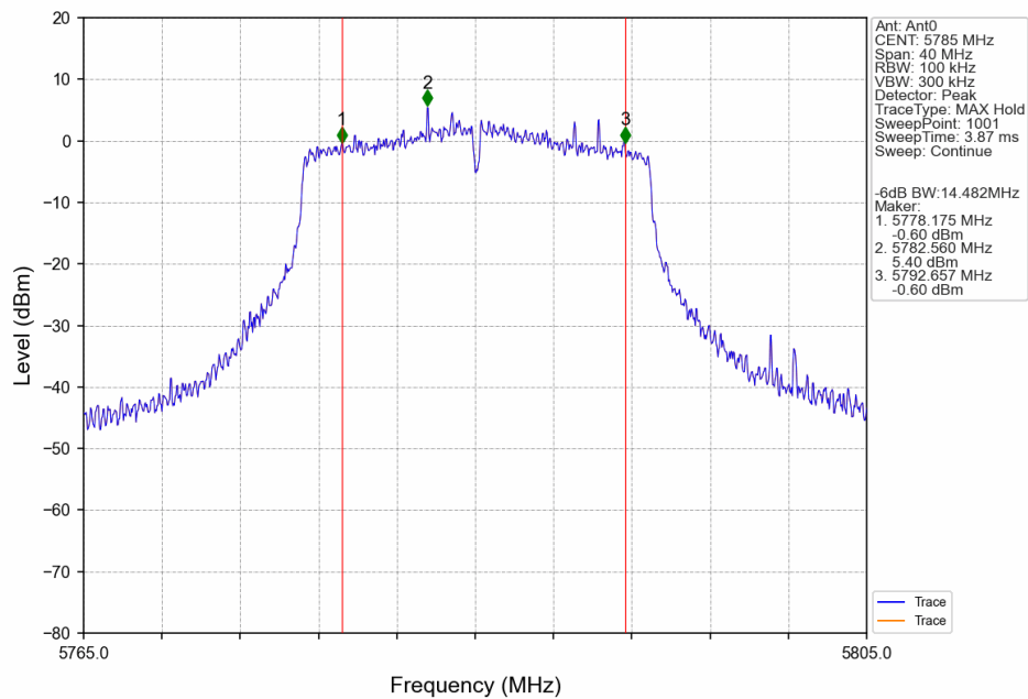
802.11ac(VHT20)_MCH_5785MHz_Ant0_NTNV
