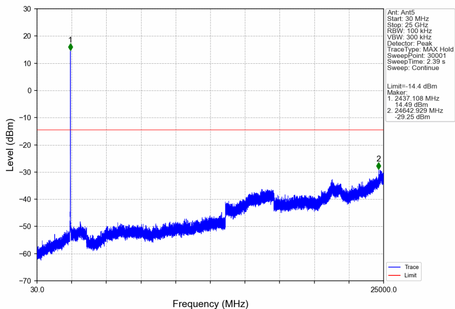
10M_MCH_2437.5MHz_Ant5_NTNV
