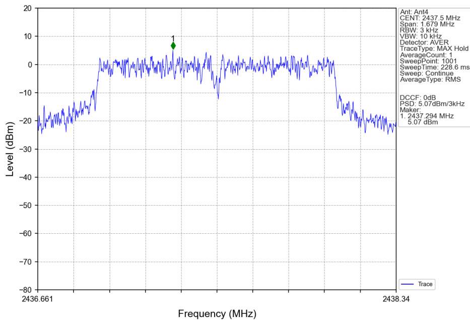
1.4M_MCH_2437.5MHz_Ant4_NTNV
