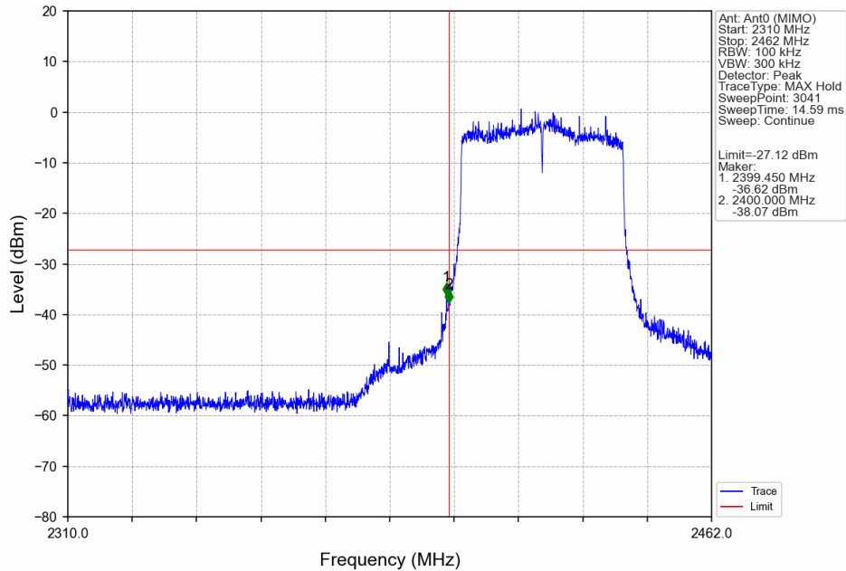
802.11ax(HEW40)_LCH_2422MHz_SU_/_Ant0 (MIMO)_NTNV
