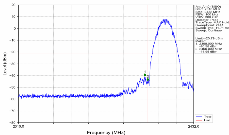
802.11b_LCH_2412MHz_Ant0 (SISO)_NTNV
