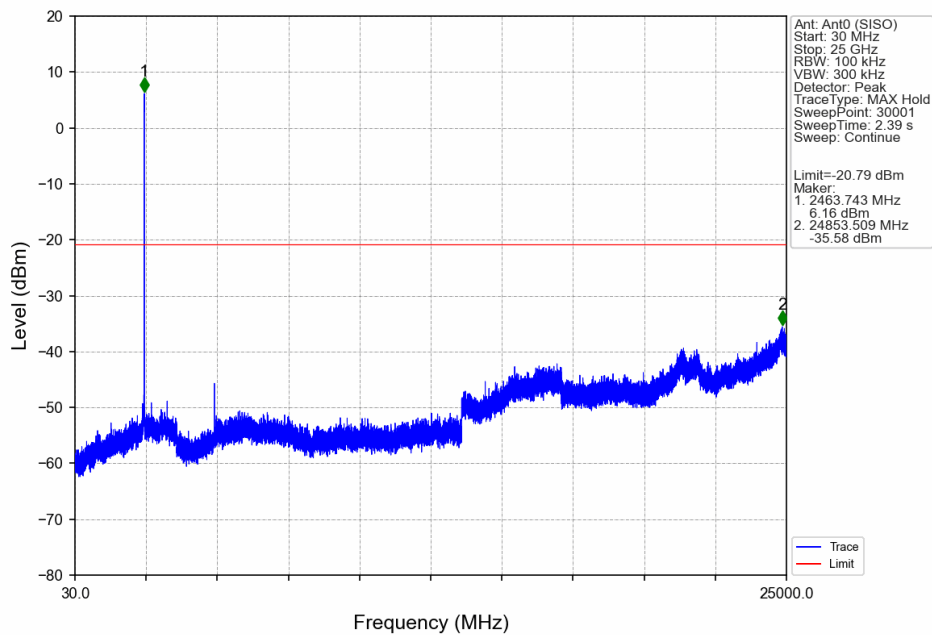
802.11b_HCH_2462MHz_Ant0 (SISO)_NTNV
