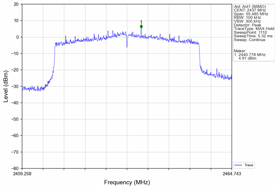
802.11ax(HEW40)_MCH_2437MHz_SU_/_Ant1 (MIMO)_NTNV
