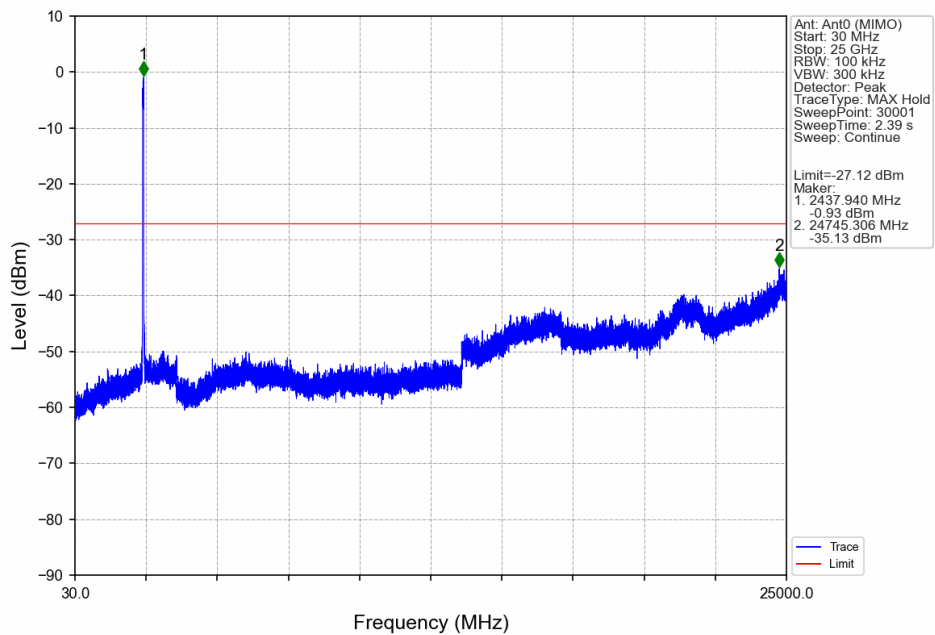
802.11ax(HEW40)_LCH_2422MHz_SU_/_Ant0 (MIMO)_NTNV
