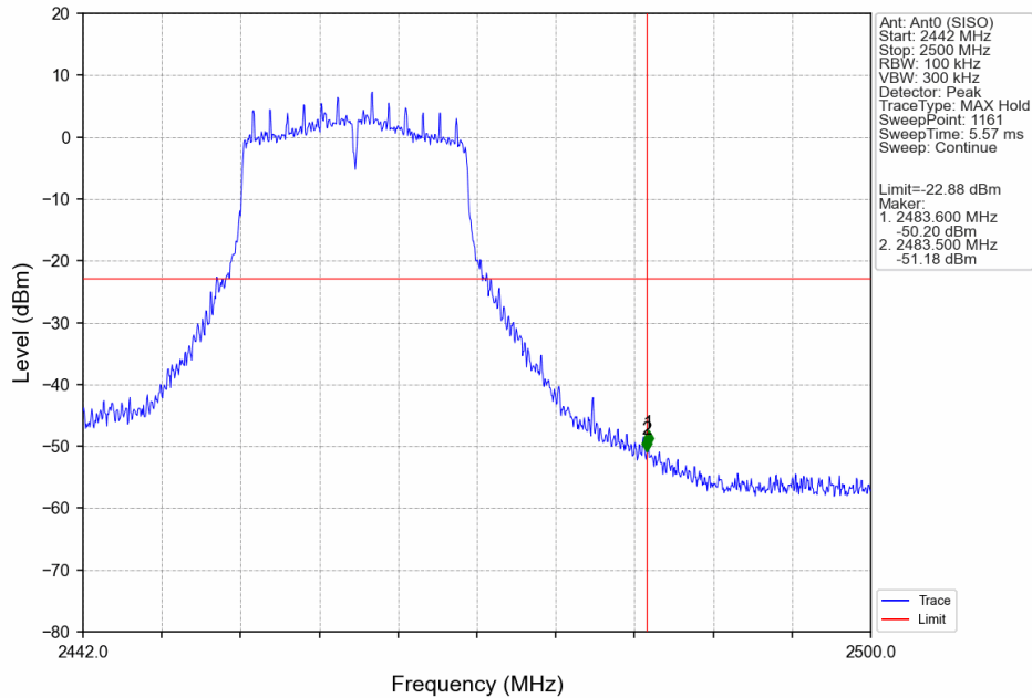
802.11g_HCH_2462MHz_Ant0 (SISO)_NTNV
