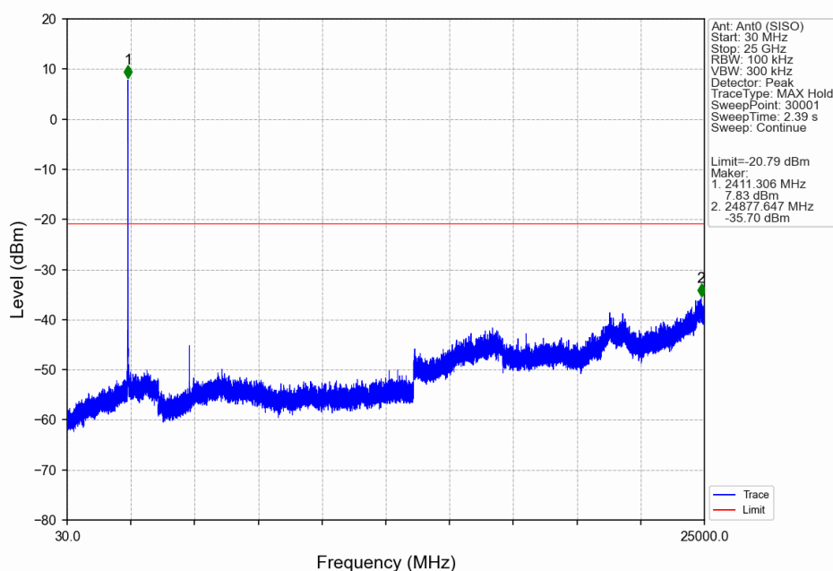
802.11b_LCH_2412MHz_Ant0 (SISO)_NTNV
