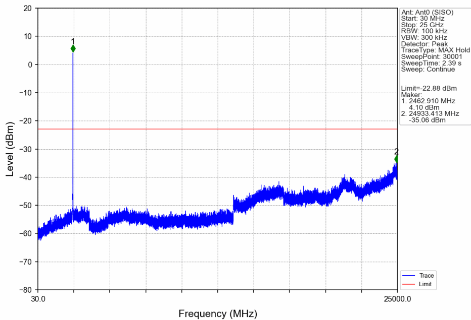
802.11g_HCH_2462MHz_Ant0 (SISO)_NTNV
