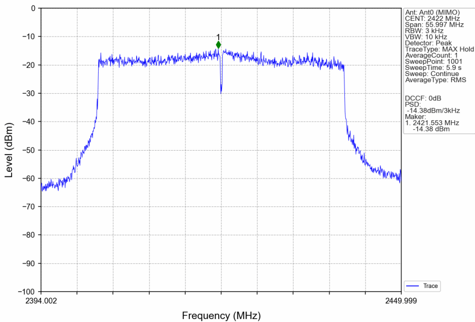
802.11ax(HEW40)_LCH_2422MHz_SU_/_Ant0 (MIMO)_NTNV
