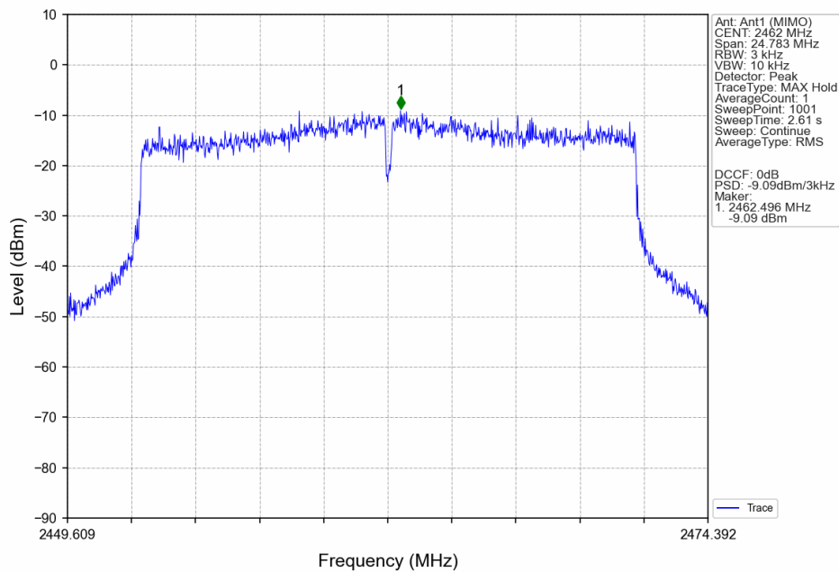
802.11ax(HEW20)_HCH_2462MHz_SU_/_Ant1 (MIMO)_NTNV
