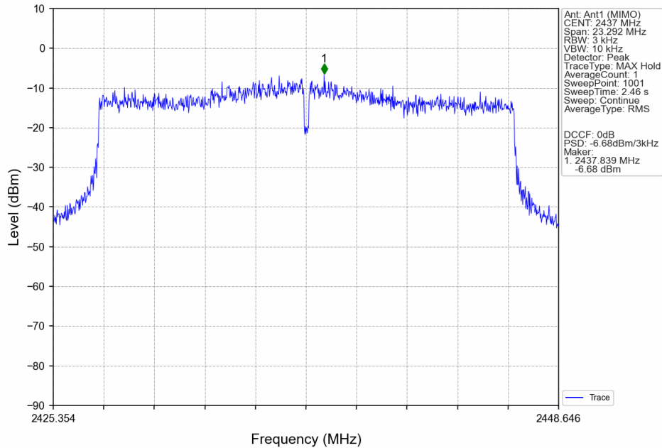
802.11ax(HEW20)_MCH_2437MHz_SU_/_MIMO_NTNV
