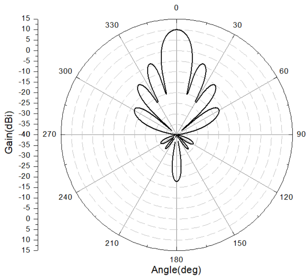
b) H 面
