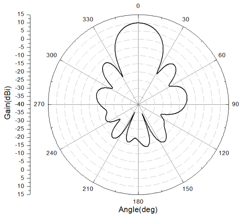
a) E 面
