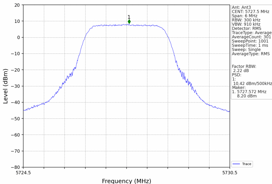
3M_LCH_5727.5MHz_MIMO_NTNV
