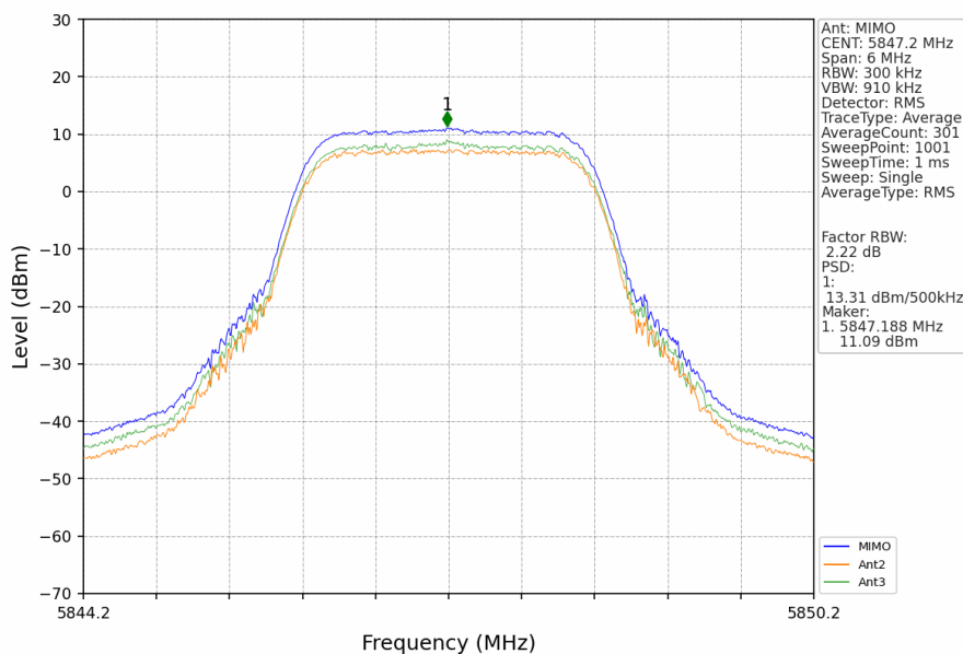
3M_HCH_5847.2MHz_MIMO_NTNV
