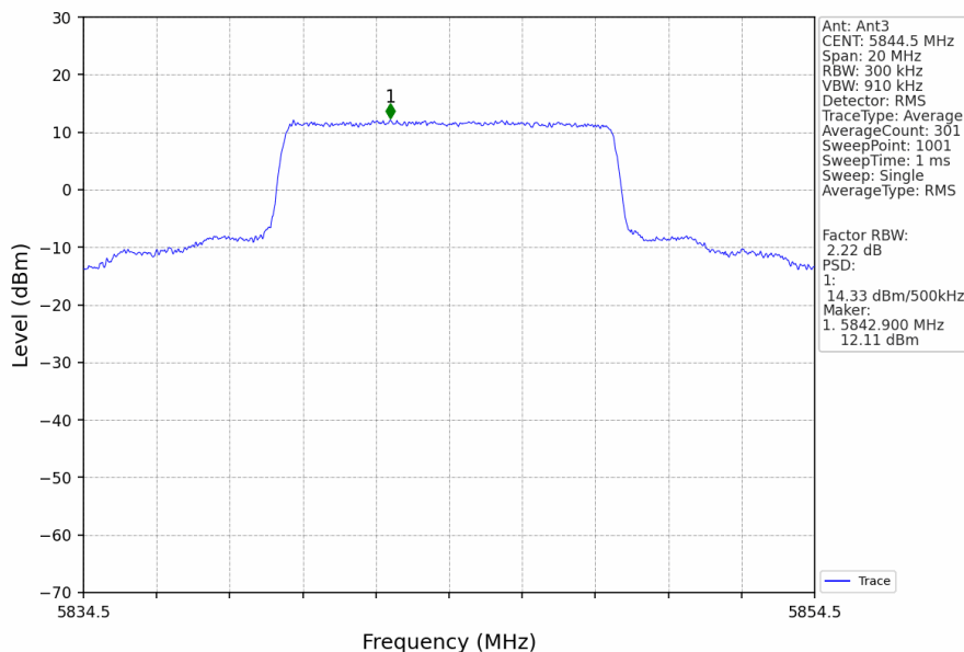
10M_HCH_5844.5MHz_MIMO_NTNV
