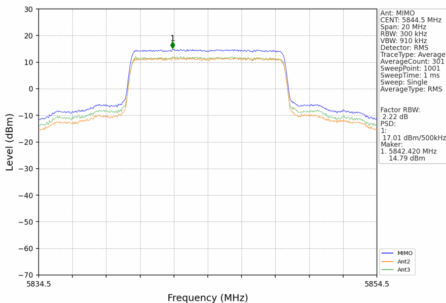
10M_HCH_5844.5MHz_MIMO_NTNV
