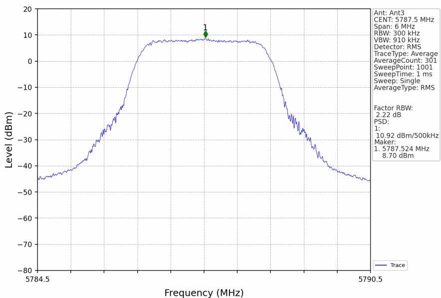
3M_MCH_5787.5MHz_Ant3_NTNV
