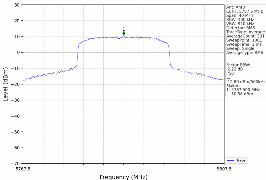
20M_MCH_5787.5MHz_MIMO_NTNV
