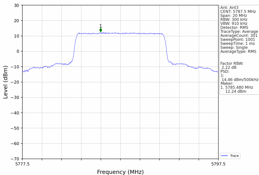
10M_MCH_5787.5MHz_Ant3_NTNV
