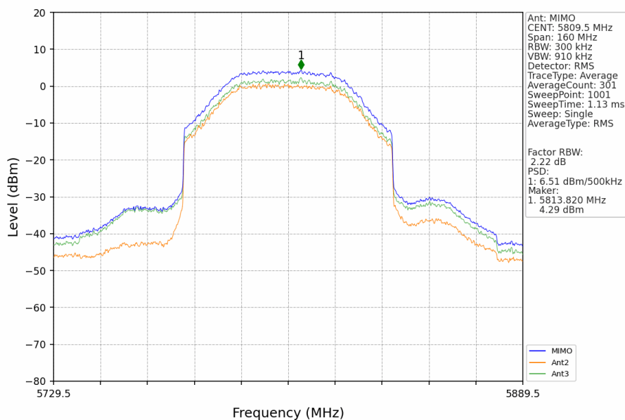
80M_HCH_5809.5MHz_MIMO_NTNV
