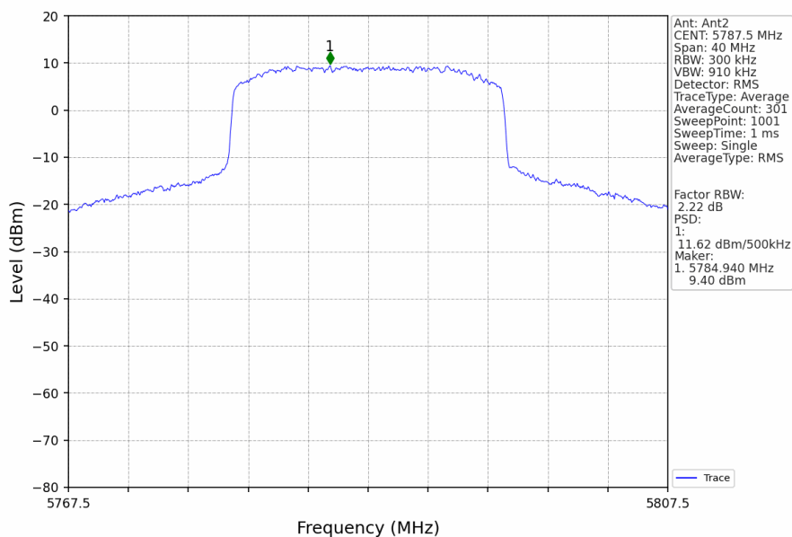
20M_MCH_5787.5MHz_Ant2_NTNV
