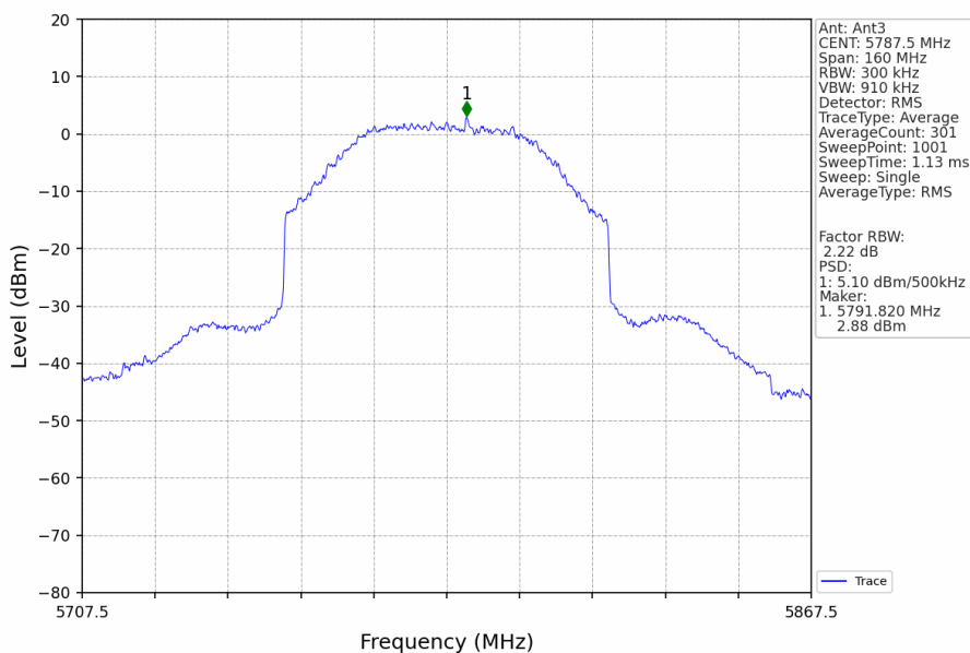
80M_MCH_5787.5MHz_Ant3_NTNV
