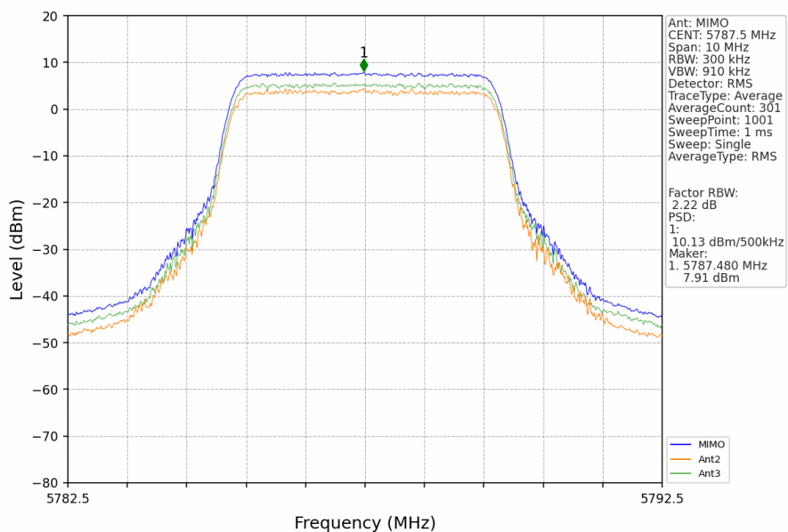
5M_MCH_5787.5MHz_MIMO_NTNV
