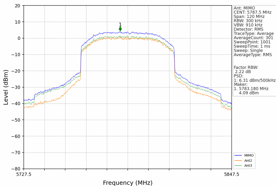
60M_MCH_5787.5MHz_MIMO_NTNV
