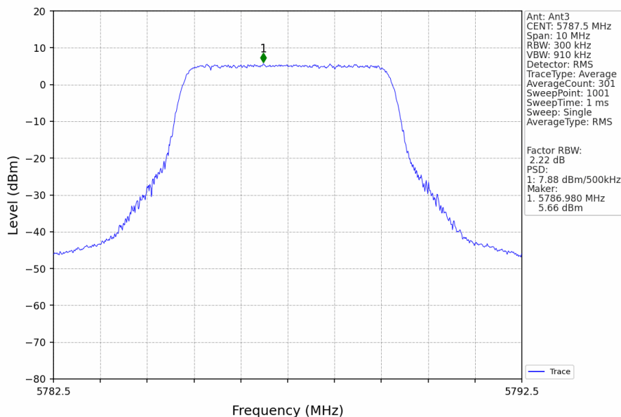
5M_MCH_5787.5MHz_MIMO_NTNV
