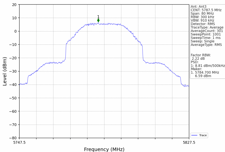
40M_MCH_5787.5MHz_Ant3_NTNV
