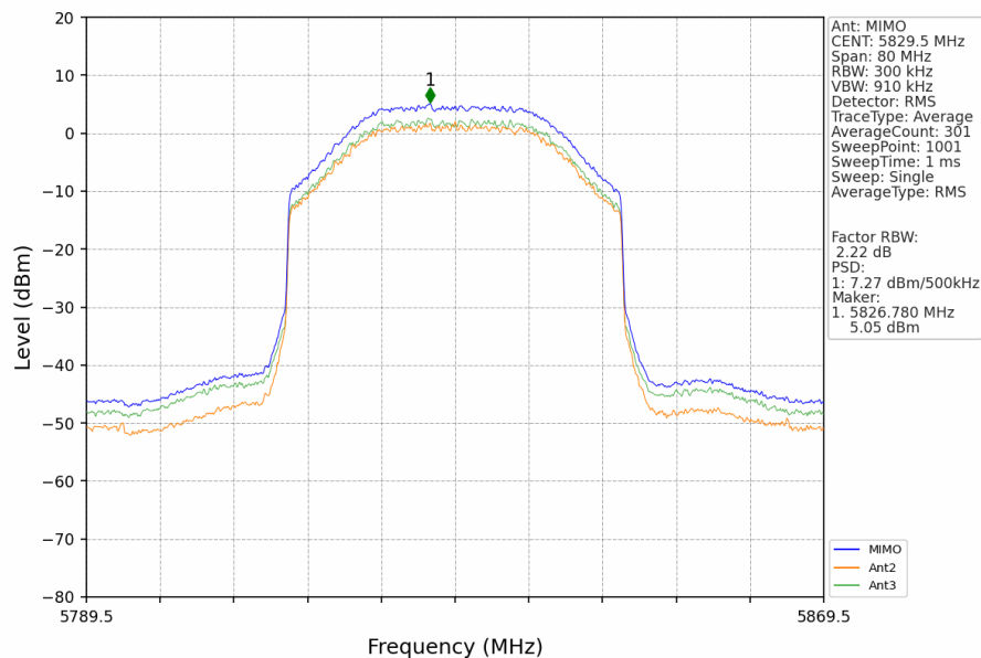
40M_HCH_5829.5MHz_MIMO_NTNV
