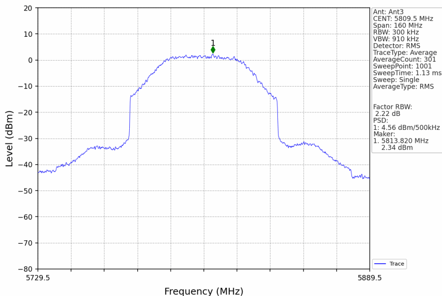
80M_HCH_5809.5MHz_MIMO_NTNV
