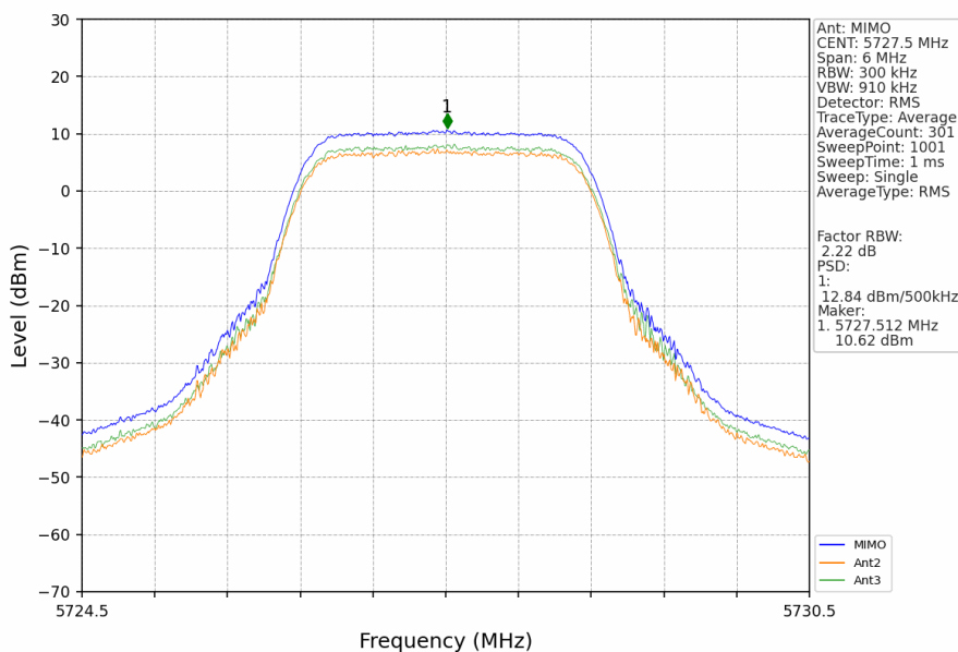
3M_LCH_5727.5MHz_MIMO_NTNV
