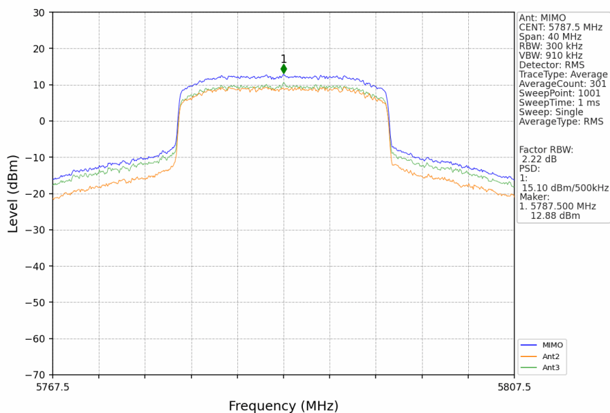
20M_MCH_5787.5MHz_MIMO_NTNV
