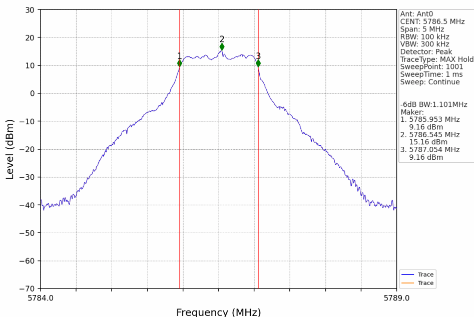
1.4M_MCH_5786.5MHz_Ant0_NTNV
