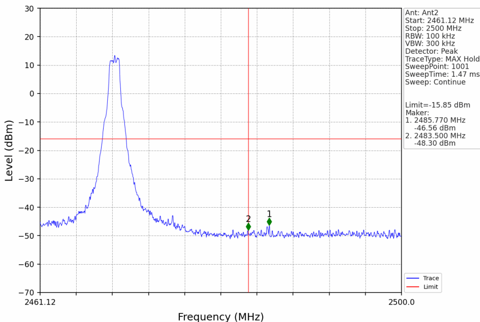
1.4M_HCH_2469.12MHz_Ant2_NTNV
