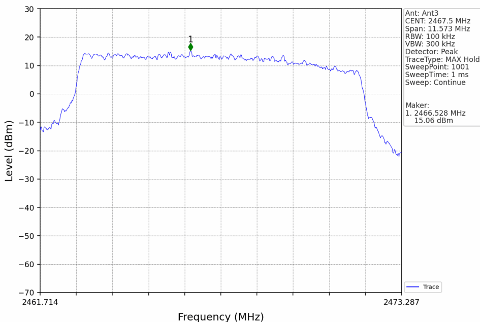
10M_HCH_2467.5MHz_Ant3_NTNV
