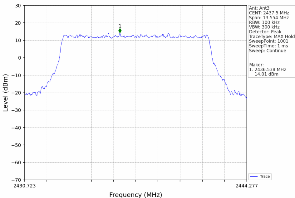
10M_MCH_2437.5MHz_Ant3_NTNV
