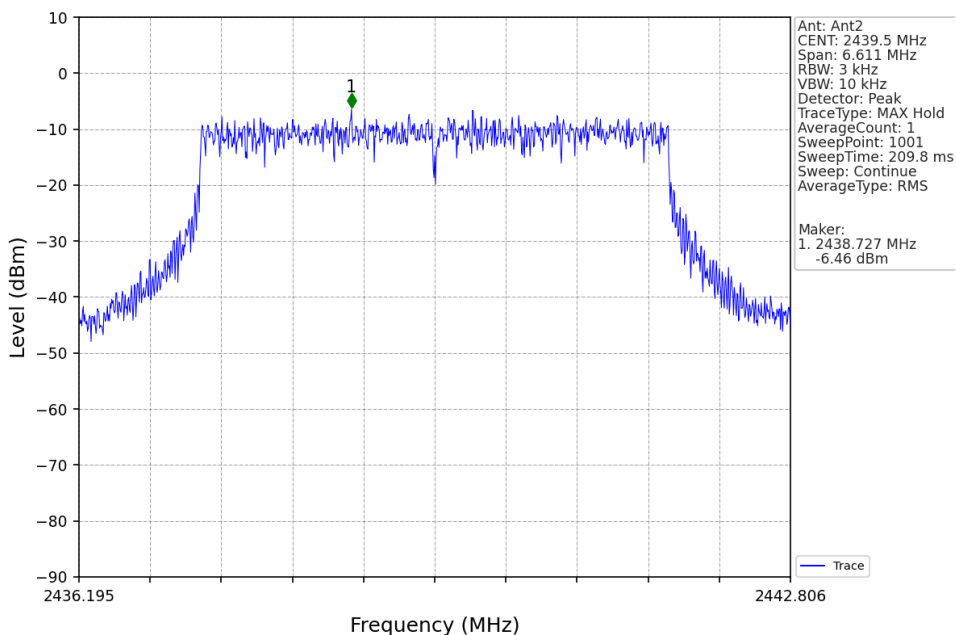
5M_MCH_2439.5MHz_Ant2_NTNV
