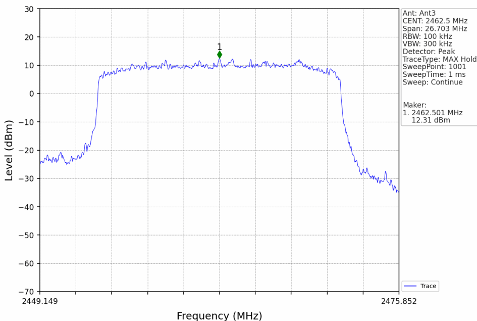
20M_HCH_2462.5MHz_Ant3_NTNV
