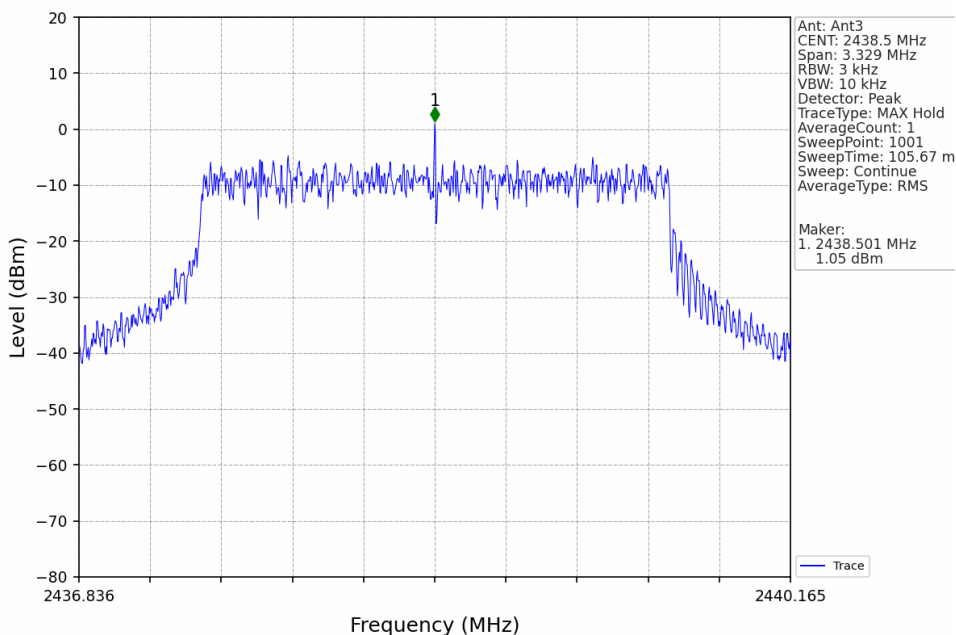
3M_MCH_2438.5MHz_Ant3_NTNV
