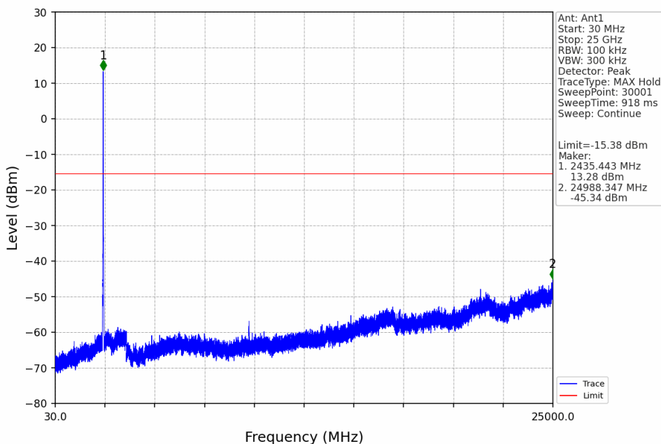
10M_MCH_2437.5MHz_Ant1_NTNV
