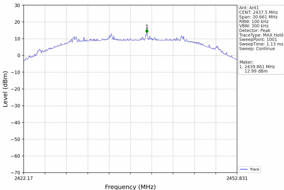
40M_MCH_2437.5MHz_Ant1_NTNV
