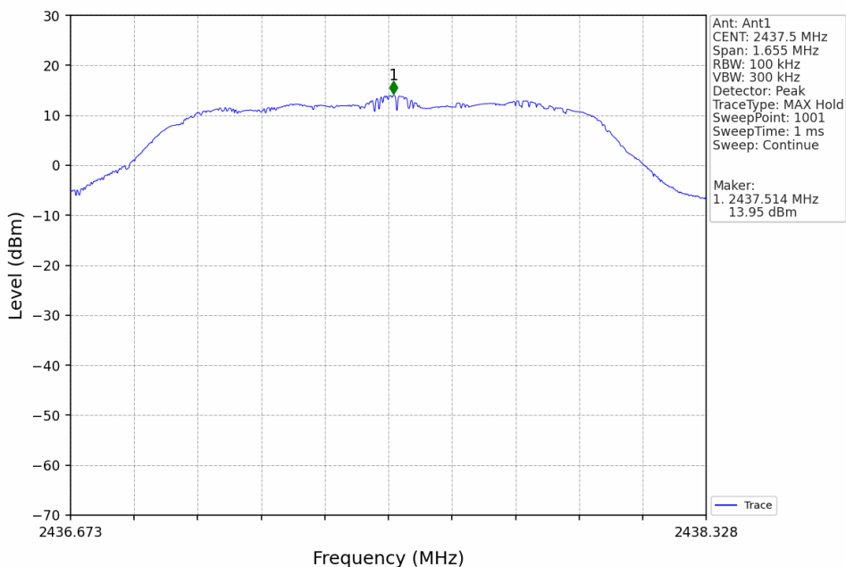
1.4M_MCH_2437.5MHz_Ant1_NTNV
