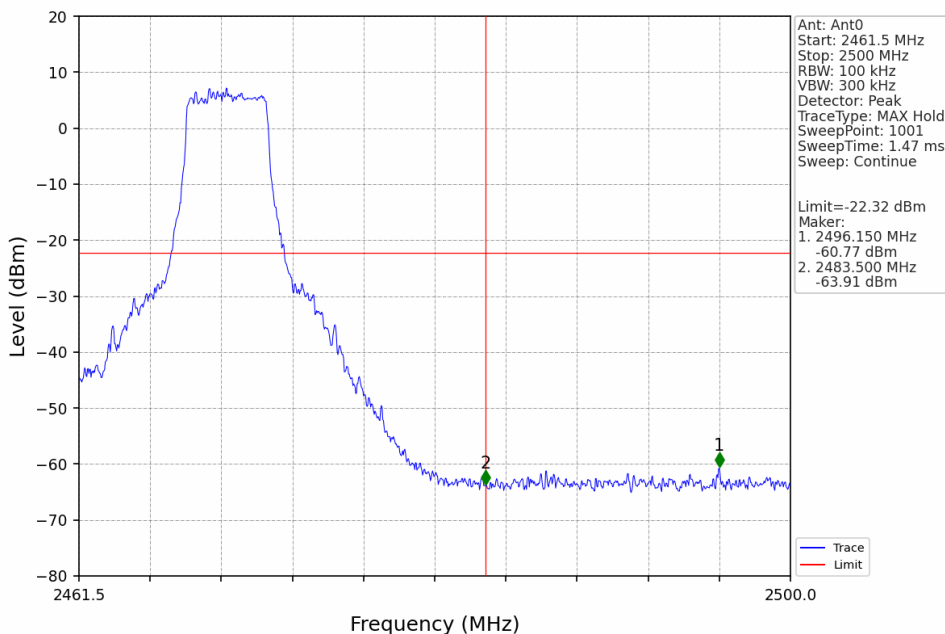
5M_HCH_2469.5MHz_Ant0_NTNV
