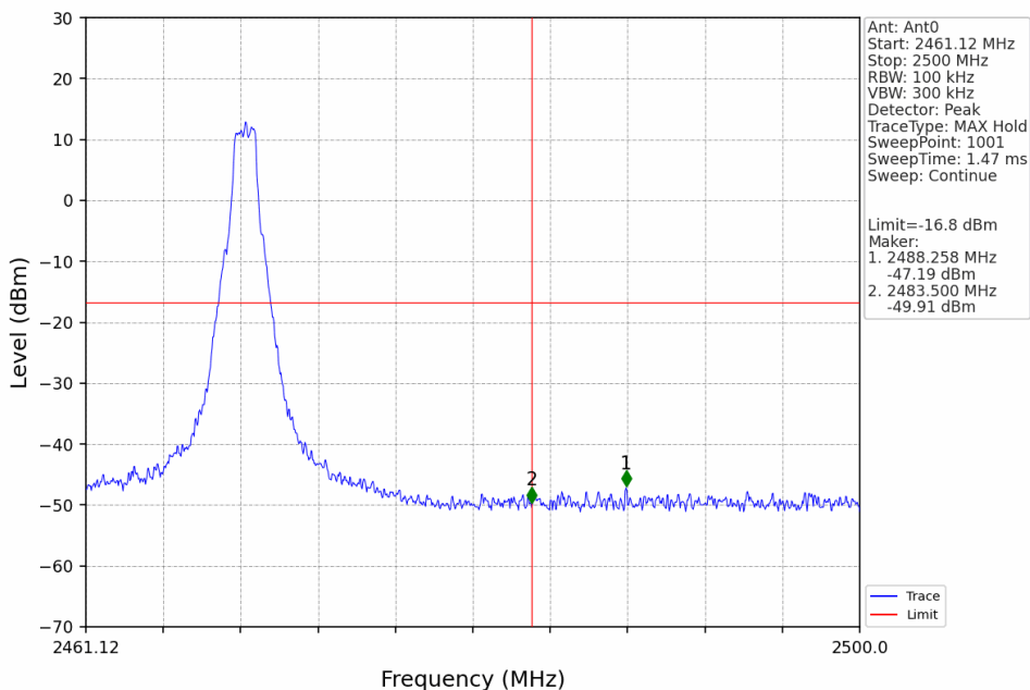
1.4M_HCH_2469.12MHz_Ant0_NTNV
