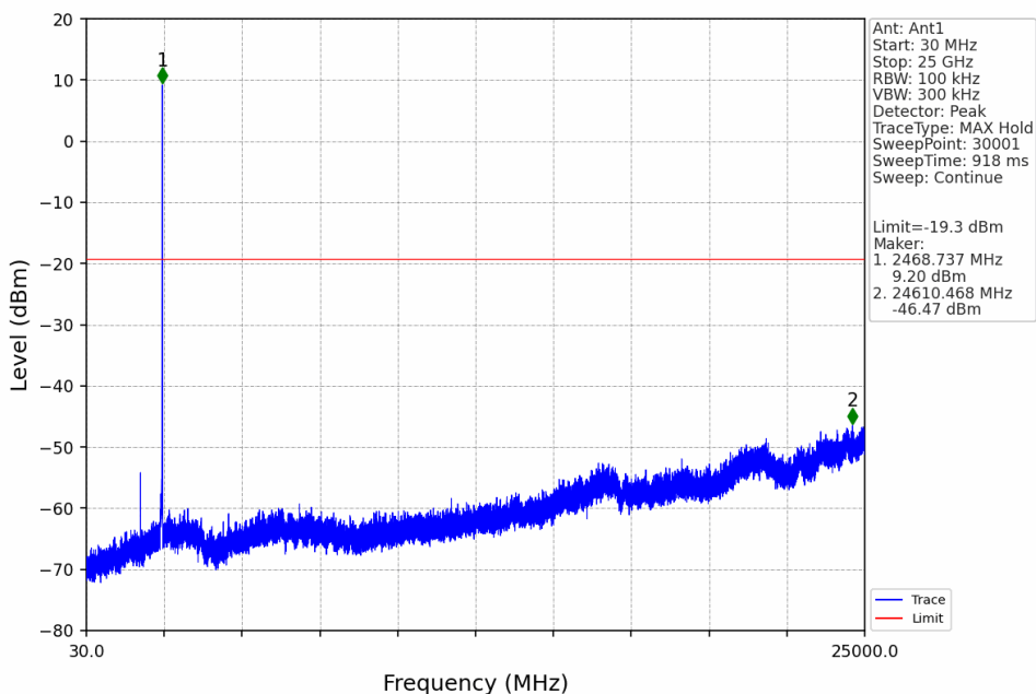
3M_HCH_2468.2MHz_Ant1_NTNV
