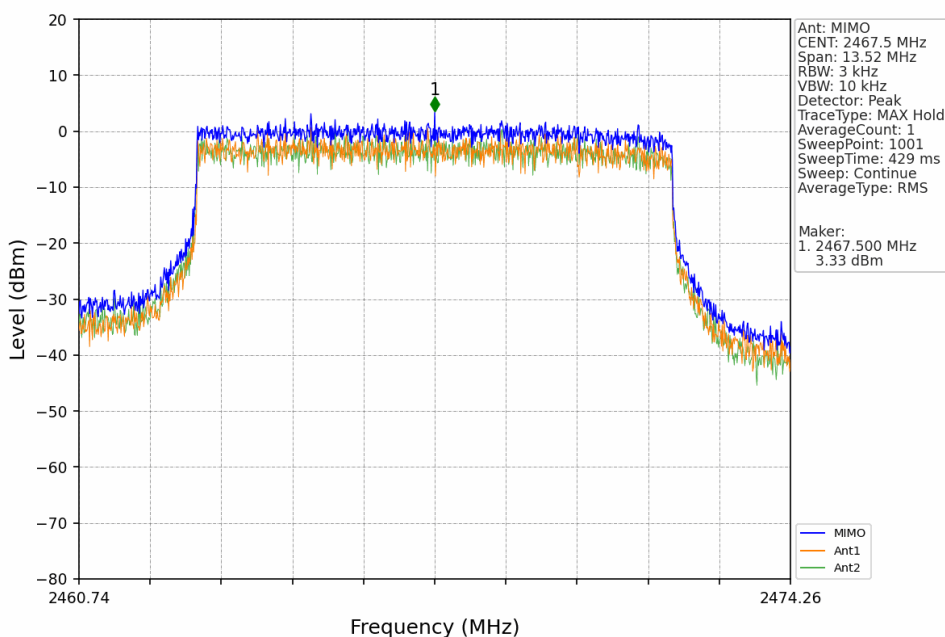
10M_HCH_2467.5MHz_MIMO_NTNV
