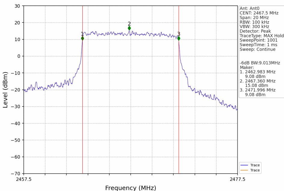
10M_HCH_2467.5MHz_Ant0_NTNV
