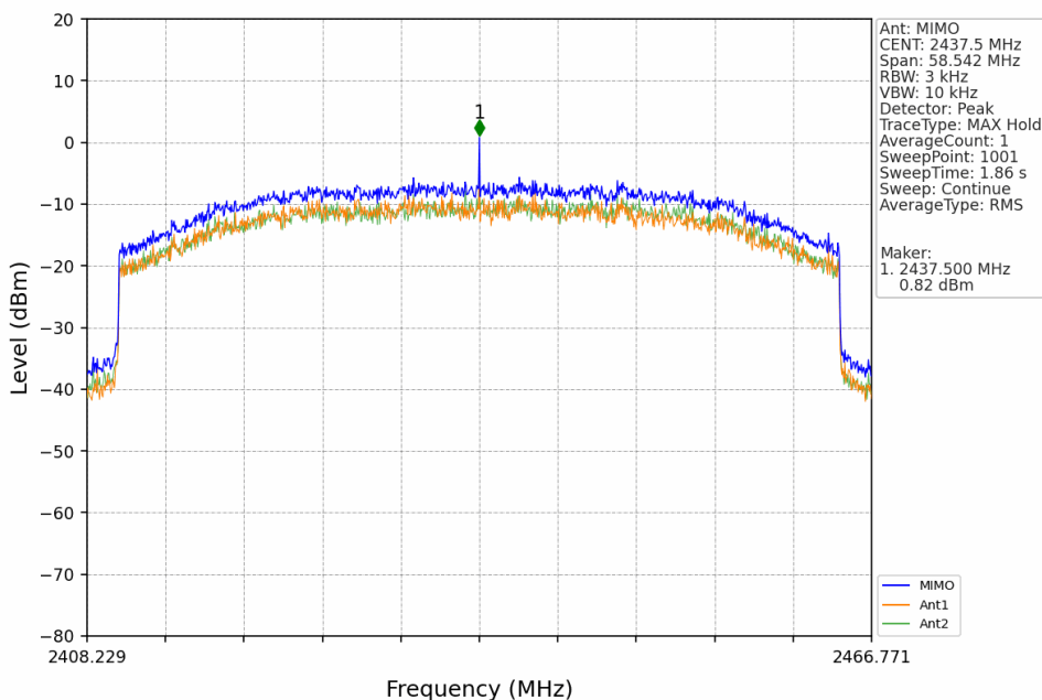
60M_MCH_2437.5MHz_MIMO_NTNV
