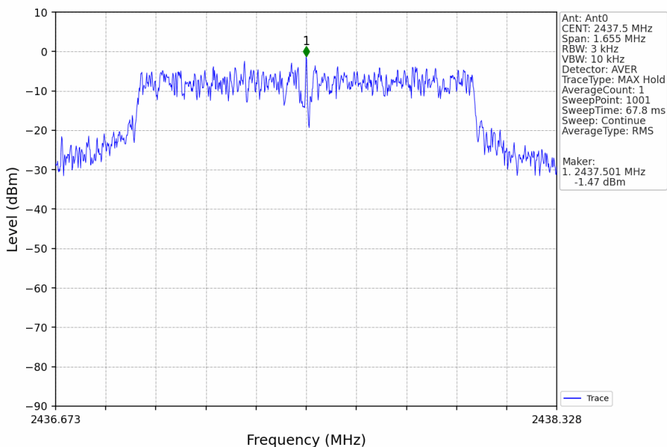
1.4M_MCH_2437.5MHz_Ant0_NTNV
