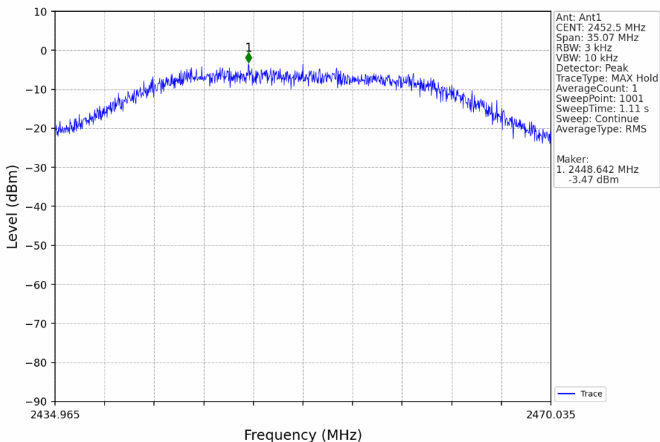
40M_HCH_2452.5MHz_MIMO_NTNV
