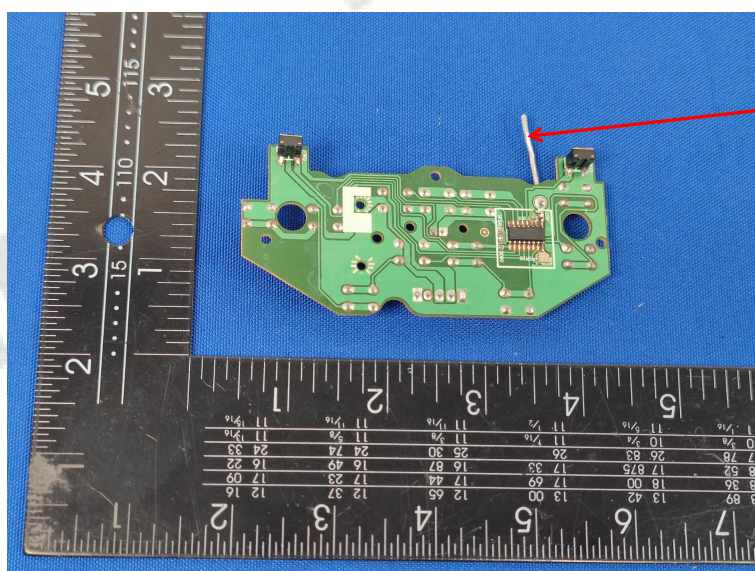
2.4GHz Antenna
