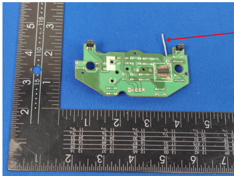
2.4GHz Antenna
