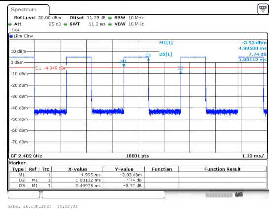
BLE 2M_Channel 0
