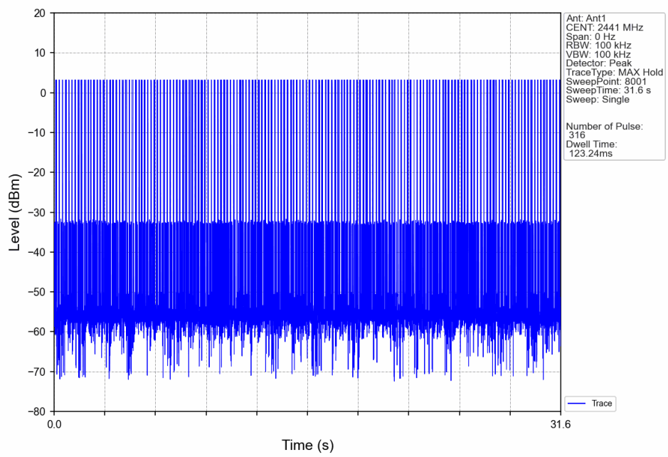
8DPSK_3DH1_HOPP_Ant1_NTNV
