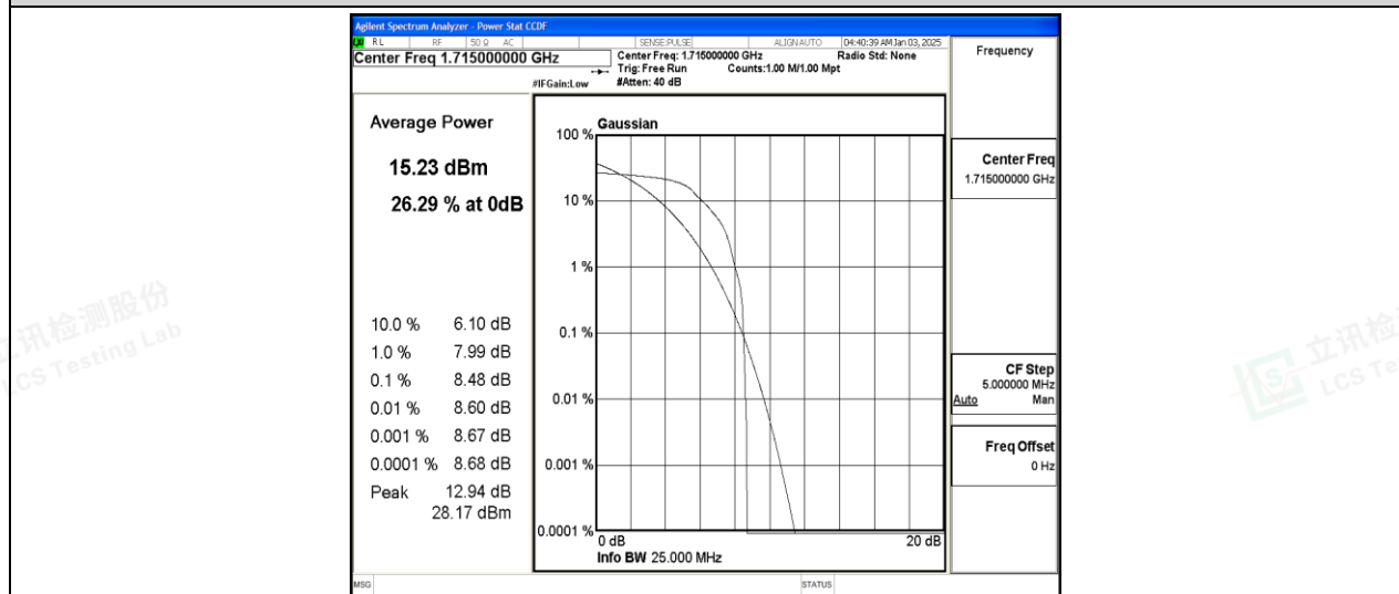
Band66-10MHz-QPSK-132022-1-0-Low-8.48-&lt;=13-PASS
