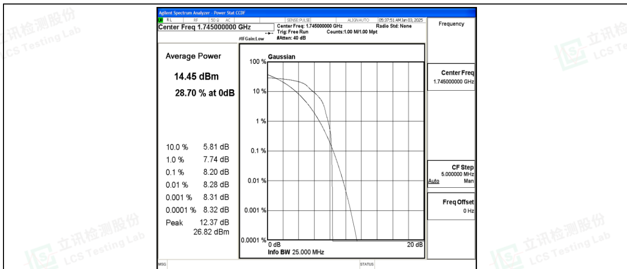
Band66-20MHz-QPSK-132322-1-0-Low-8.20-&lt;=13-PASS
