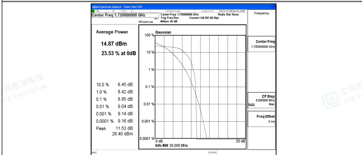
Band66-20MHz-QPSK-132072-1-0-Low-8.95-&lt;=13-PASS
