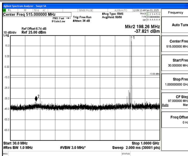
Band26-10MHz-QPSK-26740-1-0-Low-30-1000--37.82-PASS
