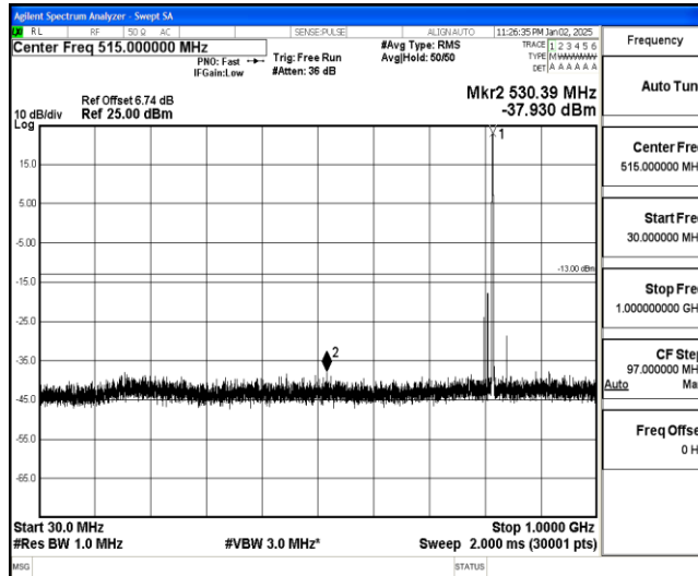
Band26-3MHz-16QAM-26740-1-0-Low-30-1000--37.93-PASS
