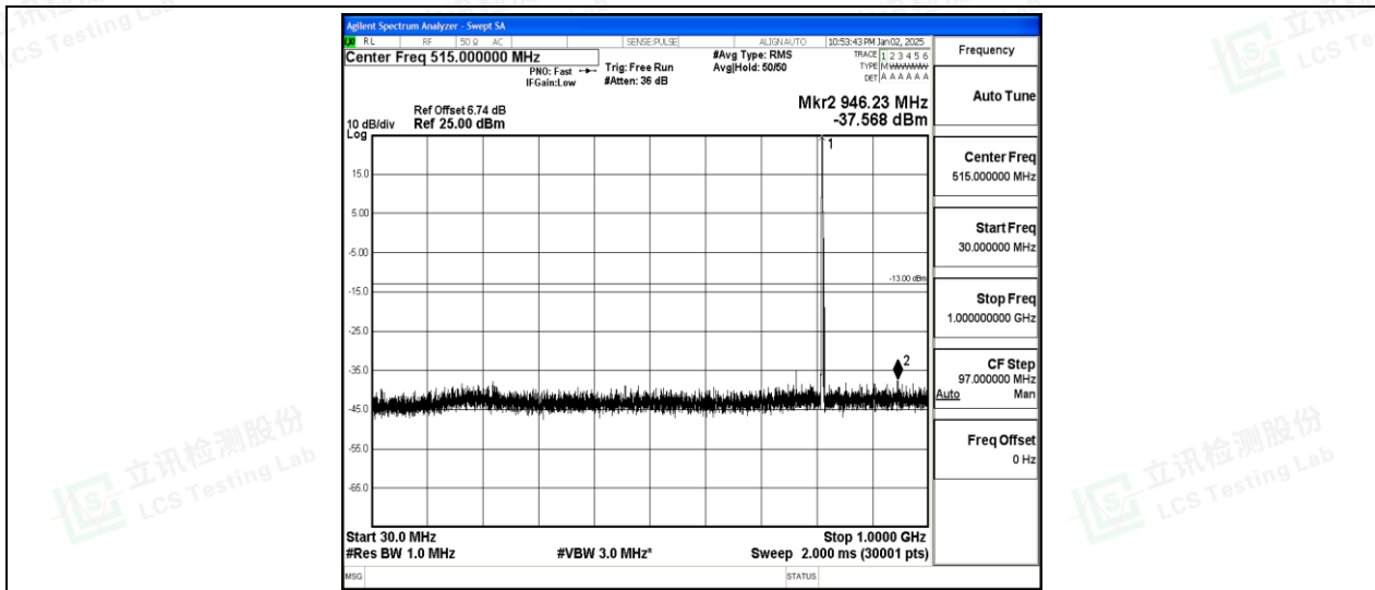
Band26-1.4MHz-QPSK-26697-1-0-Low-30-1000--37.57-PASS
