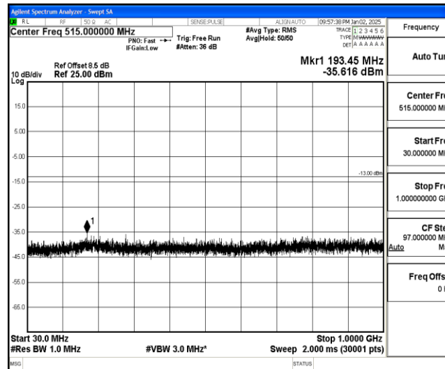
Band25-20MHz-16QAM-26365-1-0-Low-30-1000--35.62-PASS
