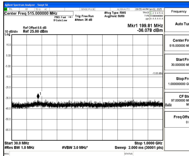
Band25-20MHz-QPSK-26365-1-0-Low-30-1000--36.08-PASS
