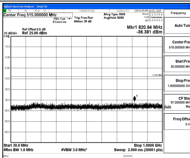
Band25-20MHz-QPSK-26140-1-0-Low-30-1000--36.38-PASS
