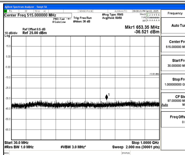
Band25-10MHz-QPSK-26090-1-0-Low-30-1000--36.52-PASS
