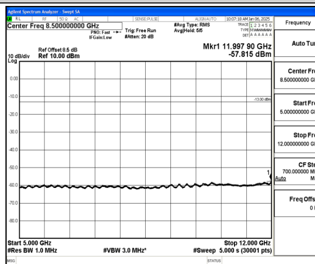
Band25-10MHz-QPSK-26365-1-0-Low-5000-12000--57.82-PASS
