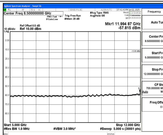
Band25-3MHz-QPSK-26365-1-0-Low-5000-12000--57.82-PASS
