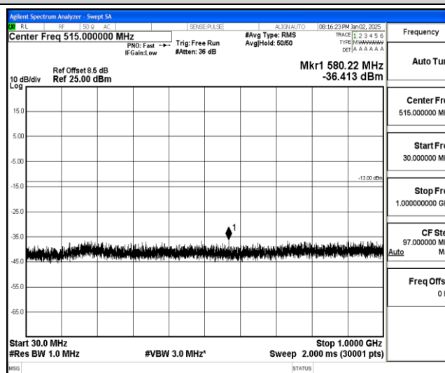
Band25-5MHz-16QAM-26065-1-0-Low-30-1000--36.41-PASS
