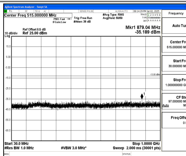
Band25-5MHz-QPSK-26065-1-0-Low-30-1000--35.19-PASS
