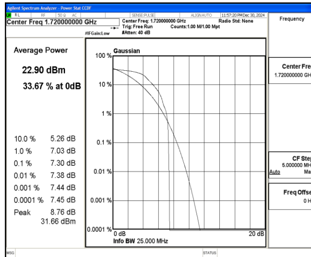
Band4-20MHz-QPSK-20050-1-0-Low-7.30-&lt;=13-PASS
