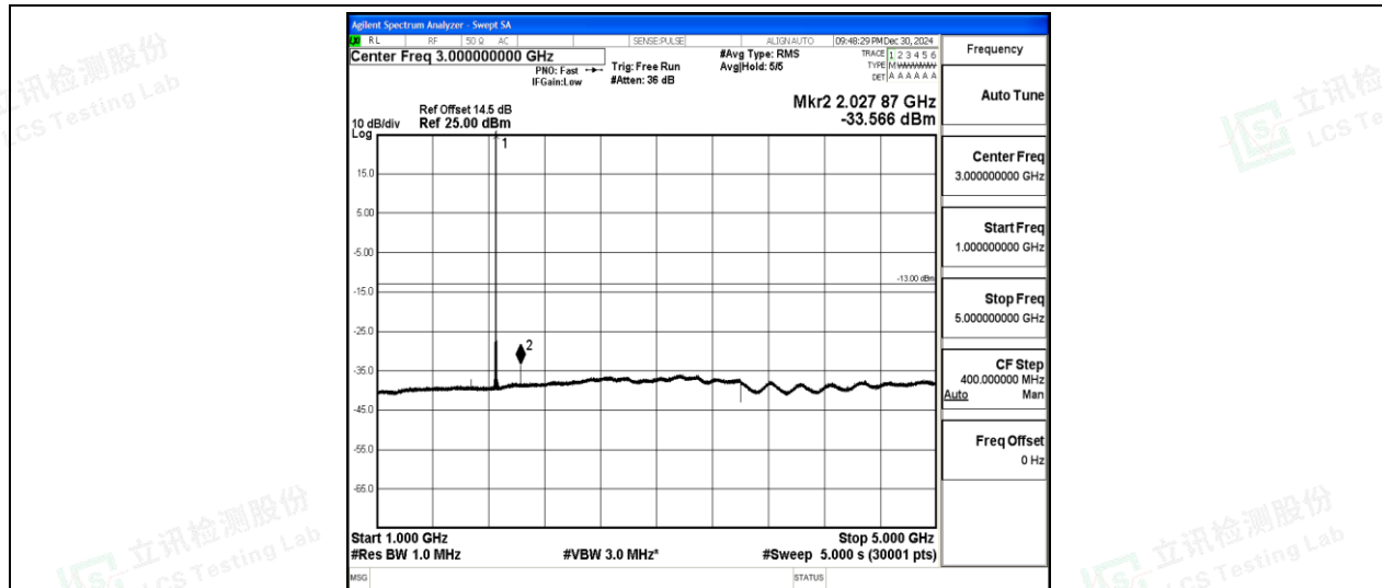
Band2-20MHz-QPSK-18700-1-0-Low-1000-5000--33.57-PASS
