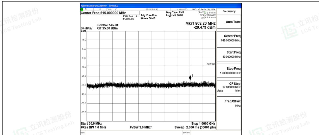
Band2-20MHz-QPSK-18900-1-0-Low-30-1000--29.47-PASS
