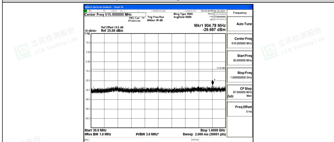
Band2-20MHz-16QAM-18700-1-0-Low-30-1000--29.69-PASS
