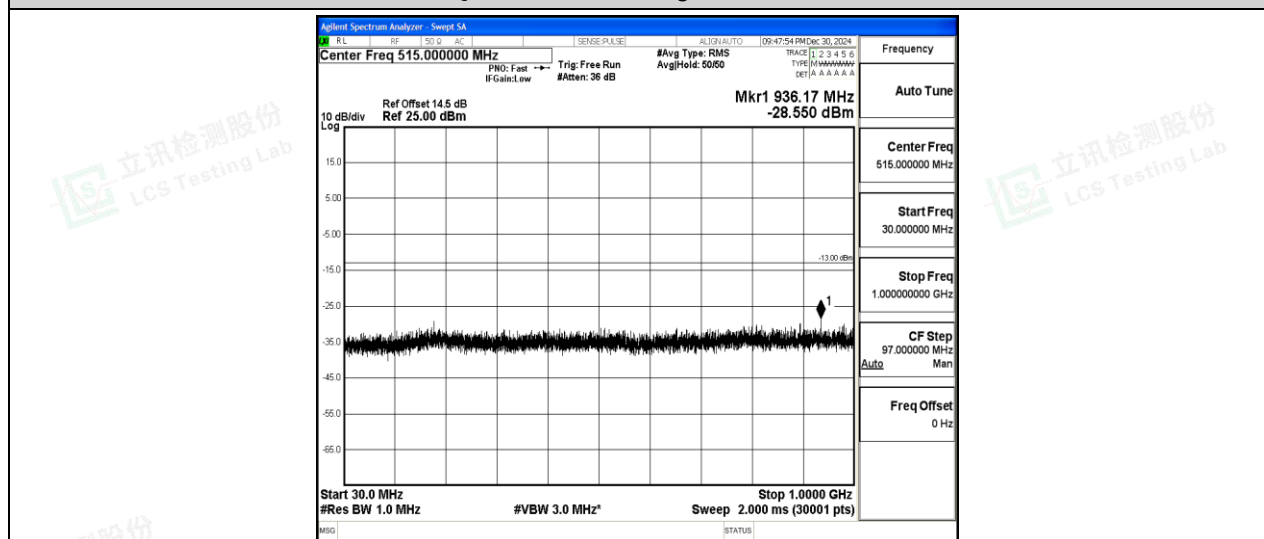
Band2-20MHz-QPSK-18700-1-0-Low-30-1000--28.55-PASS
