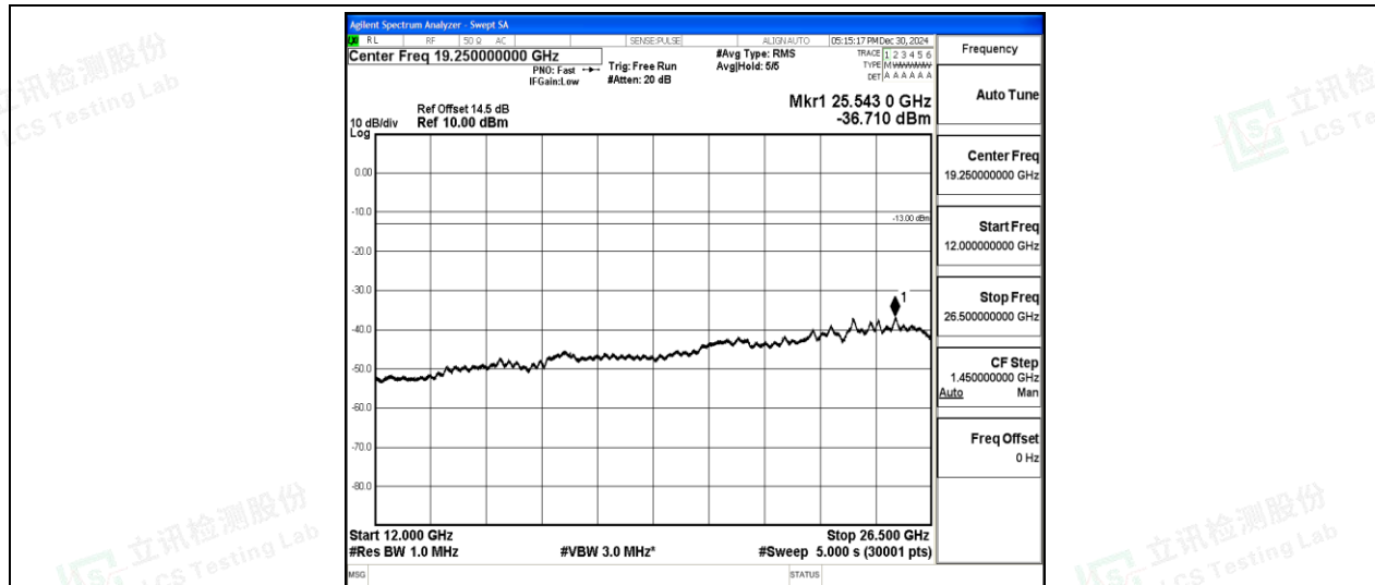
Band2-5MHz-QPSK-18900-1-0-Low-12000-26500--36.71-PASS
