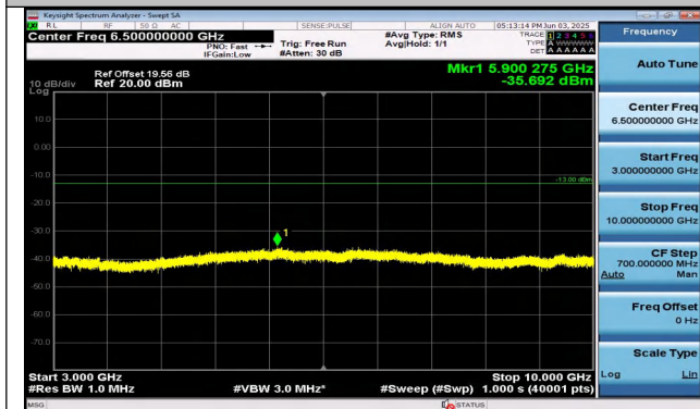
Band26(824-849)-10MHz-QPSK-26990-50RB#0-3000~10 000-PASS
