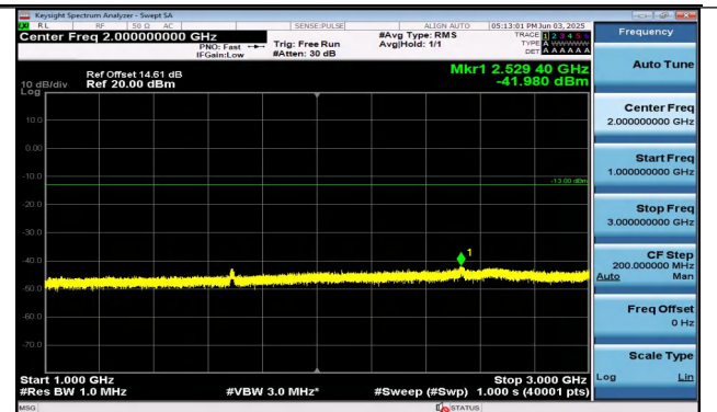
Band26(824-849)-10MHz-QPSK-26990-50RB#0-1000~30 00-PASS
