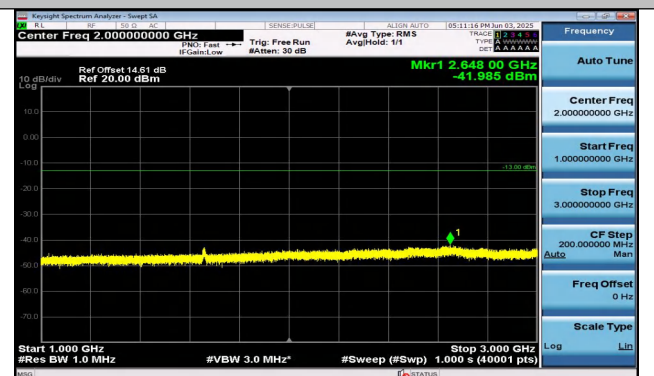
Band26(824-849)-10MHz-QPSK-26840-50RB#0-1000~3000-PASS
