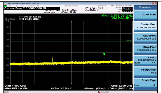
Band26(824-849)-5MHz-QPSK-27015-1RB#0-1000~3000-
