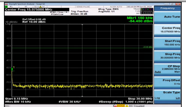
Band26(824-849)-10MHz-QPSK-26840-50RB#0-0.15~30-PASS
