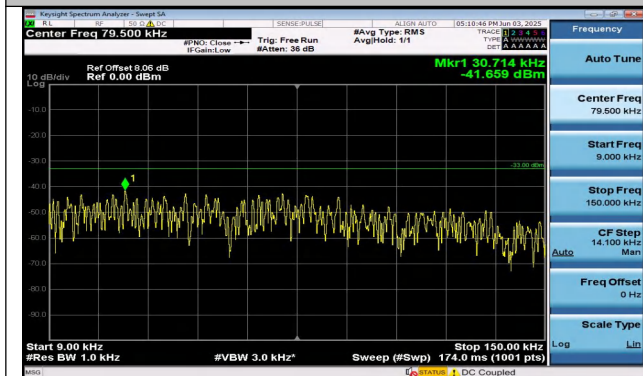
Band26(824-849)-10MHz-QPSK-26840-50RB#0-0.009~0.15-PASS
