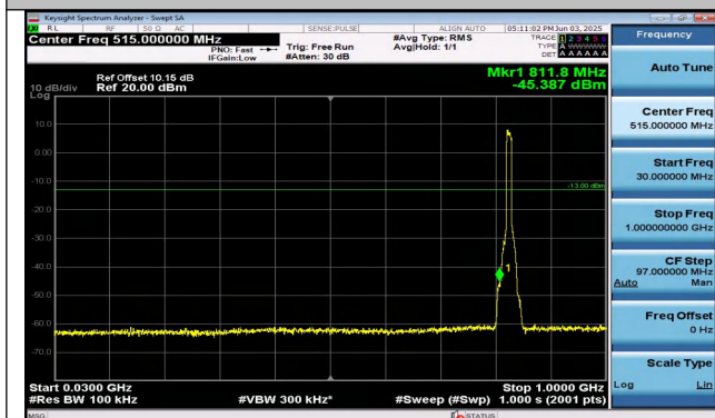
Band26(824-849)-10MHz-QPSK-26840-50RB#0-30~1000-PASS
