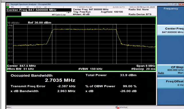
Band26(824-849)-3MHz-QPSK-27025-15RB#0-PASS
