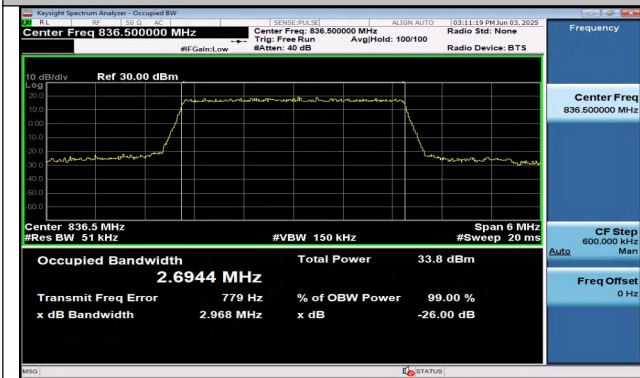
Band26(824-849)-3MHz-QPSK-26915-15RB#0-PASS
