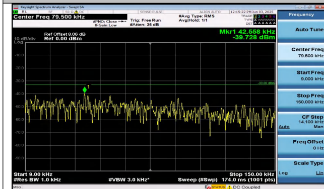
Band26(814-824)-3MHz-QPSK-26775-15RB#0-0.009~0.15 -PASS
