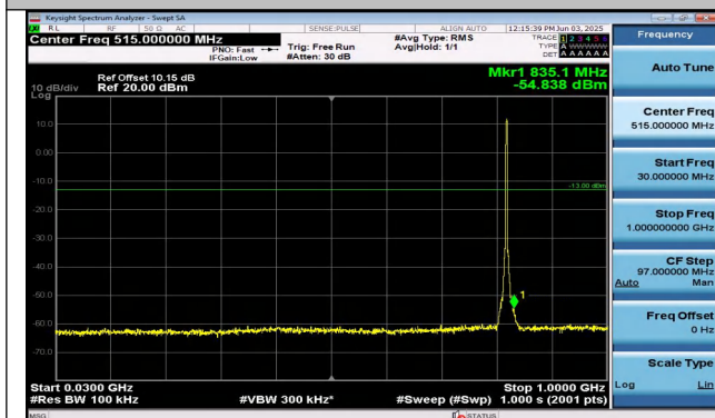
Band26(814-824)-3MHz-QPSK-26775-15RB#0-30~1000-P ASS
