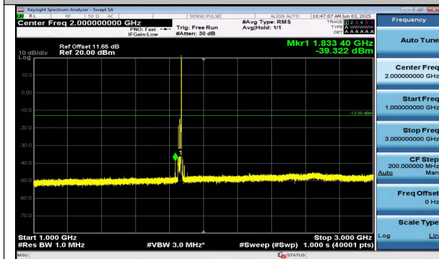
Band25-20MHz-QPSK-26140-1RB#99-1000~3000-PASS
