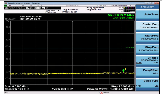
Band25-20MHz-QPSK-26365-1RB#0-30~1000-PASS
