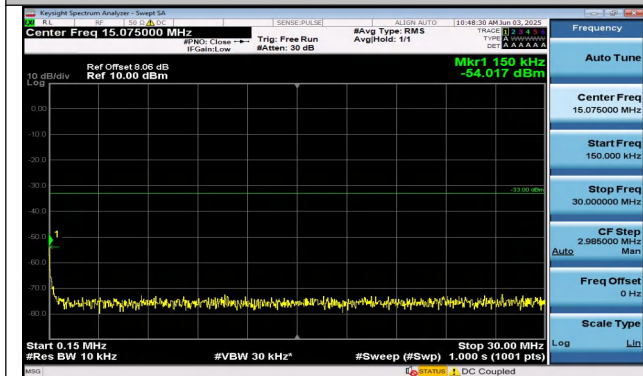
Band25-20MHz-QPSK-26365-1RB#0-0.15~30-PASS
