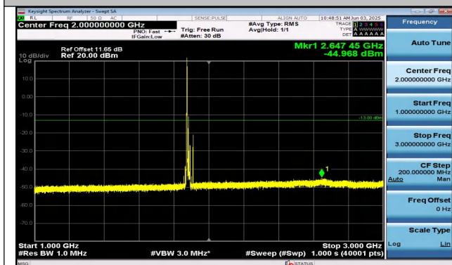
Band25-20MHz-QPSK-26365-1RB#0-1000~3000-PASS
