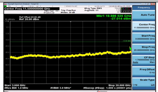
Band25-20MHz-QPSK-26365-1RB#0-3000~20000-PASS
