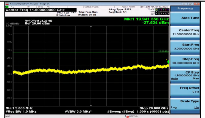
Band25-15MHz-QPSK-26115-1RB#0-3000~20000-PASS
