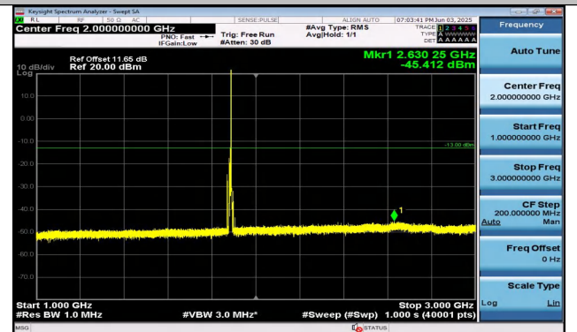
Band25-10MHz-QPSK-26365-1RB#49-1000~3000-PASS
