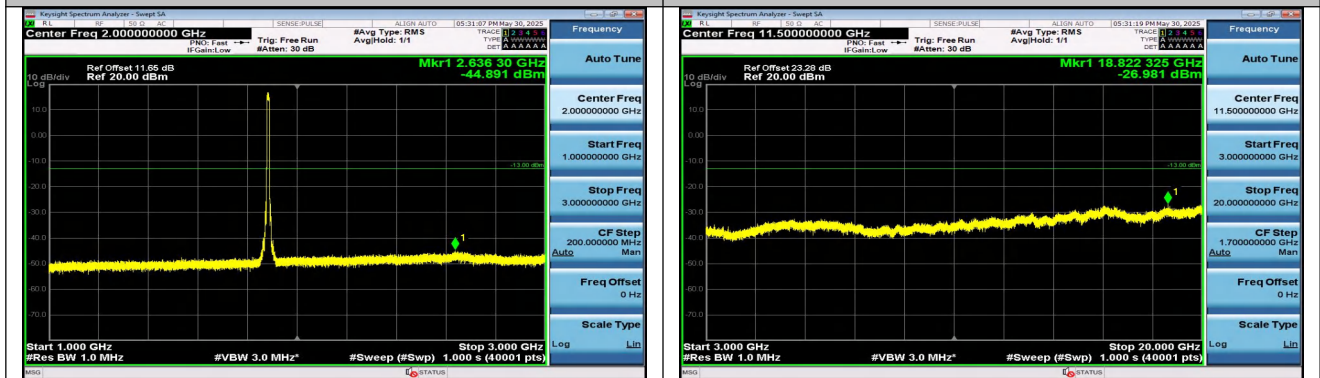
Band25-10MHz-QPSK-26365-50RB#0-1000~3000-PASS
