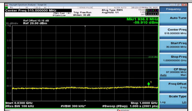
Band25-10MHz-QPSK-26365-1RB#0-30~1000-PASS
