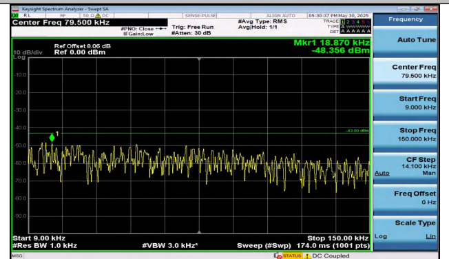
Band25-10MHz-QPSK-26365-50RB#0-0.009~0.15-PASS
