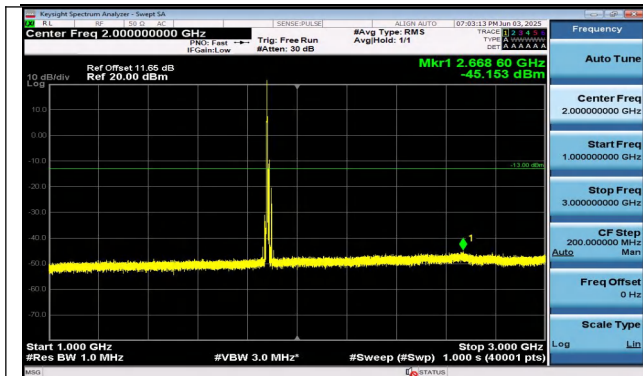
Band25-10MHz-QPSK-26365-1RB#0-1000~3000-PASS
