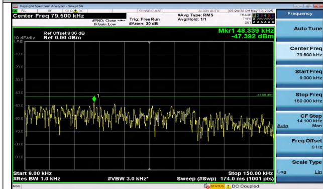
Band25-10MHz-QPSK-26365-1RB#49-0.009~0.15-PASS
