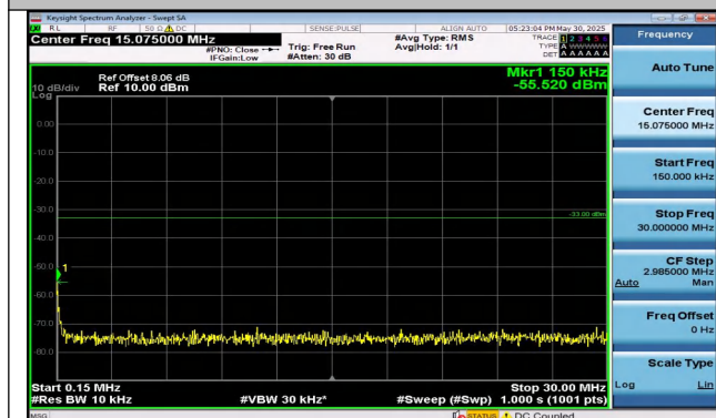
Band25-10MHz-QPSK-26365-1RB#0-0.15~30-PASS
