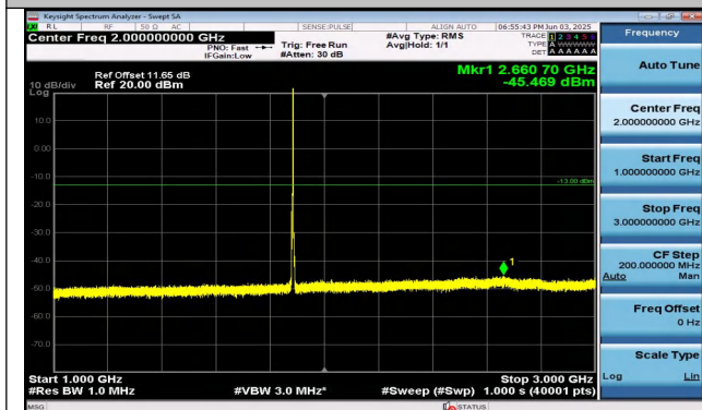
Band25-3MHz-QPSK-26365-1RB#14-1000~3000-PASS
