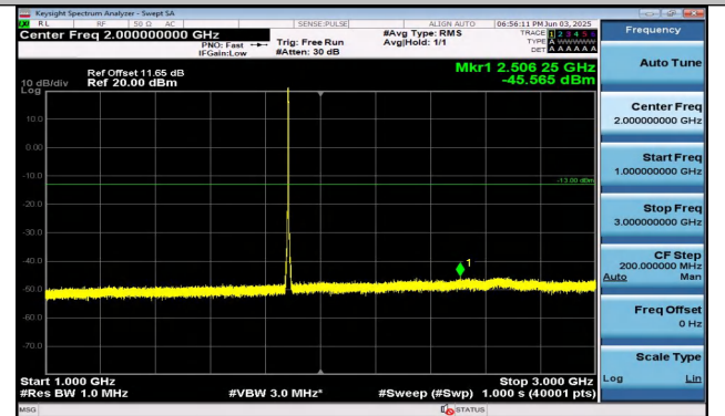
Band25-3MHz-QPSK-26365-15RB#0-1000~3000-PASS
