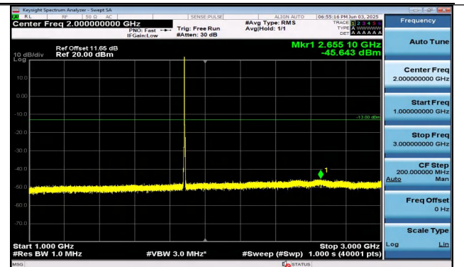
Band25-3MHz-QPSK-26365-1RB#0-1000~3000-PASS
