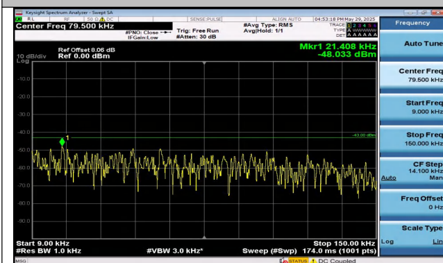
Band25-1.4MHz-QPSK-26365-6RB#0-0.009~0.15-PASS
